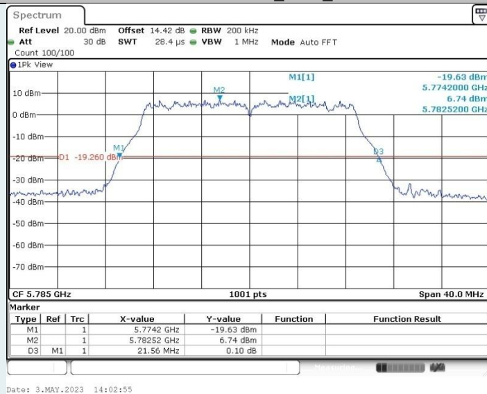
802.11ac VHT20 MIMO Ant2 5785 MHz
