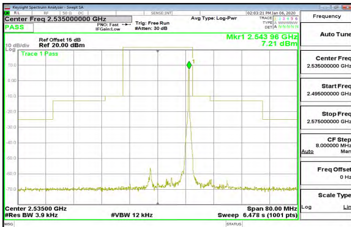
Band7_20MHz_QPSK_1_99_CH21350
