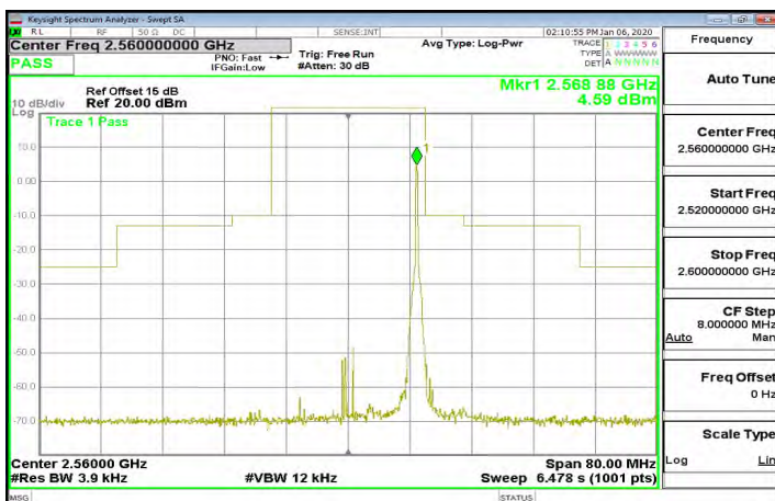
Band7_20MHz_64QAM_1_99_CH21350
