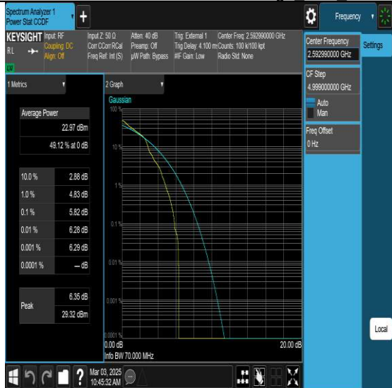
NTNV-N41-PC3-30-70-M-DFT-QPSK-Edge 1RB Left-PASS
