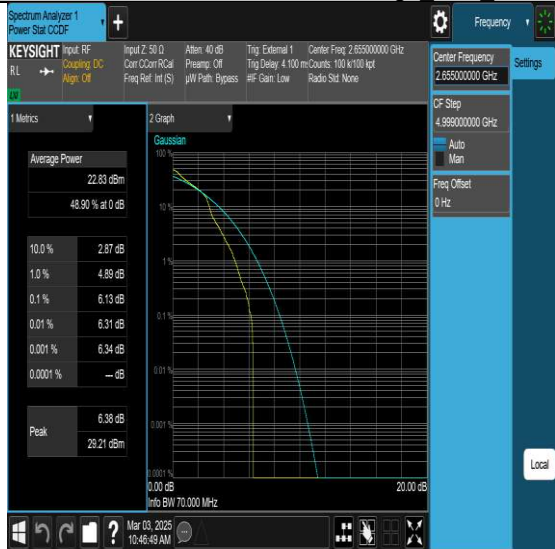
NTNV-N41-PC3-30-70-H-DFT-QPSK-Edge 1RB Left-PASS
