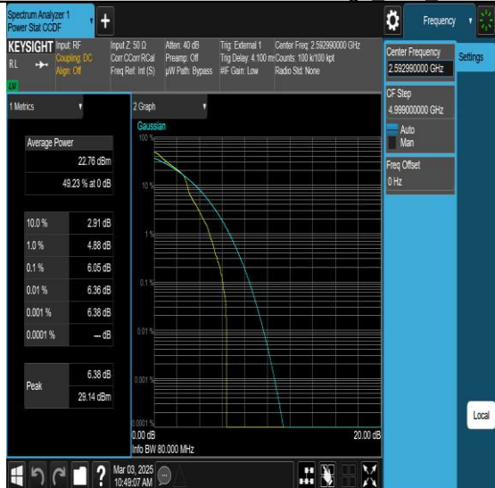
NTVN-N41-PC3-30-80-M-DFT-QPSK-Edge 1RB Left-PASS
