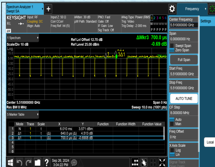
NTNV-11N40MIMO-Ant1-5510
