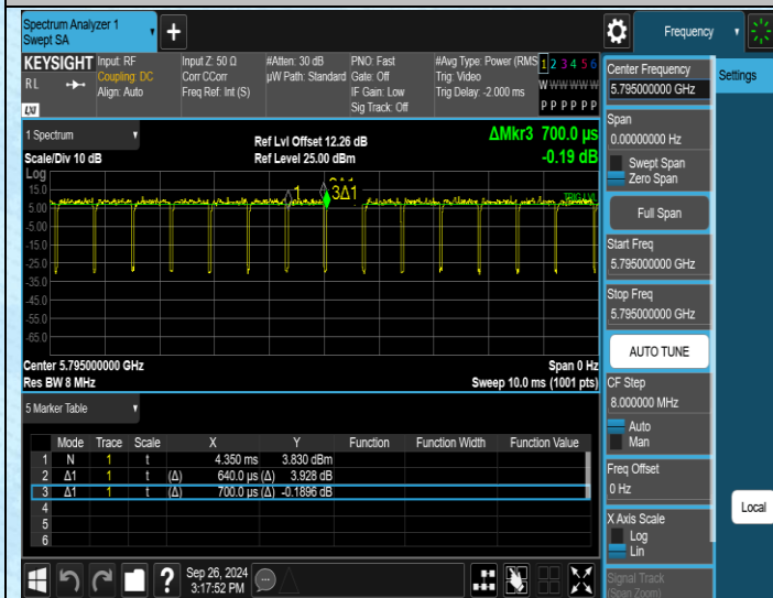
NTNV-11N40MIMO-Ant1-5795
