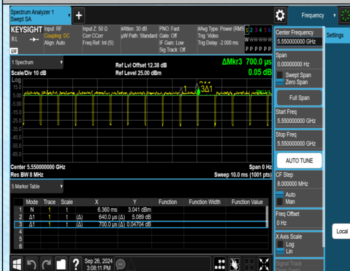
NTNV-11N40MIMO-Ant1-5550
