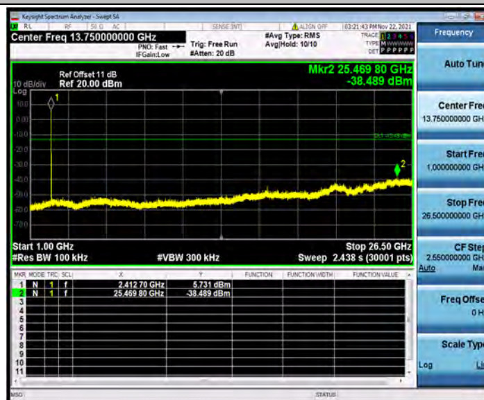
11AX20MIMO_Ant1_2412_26Tone_RU8_0~Reference
