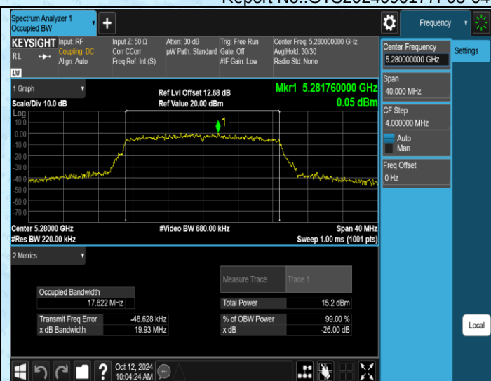
11N20MIMO-Ant2-5280
