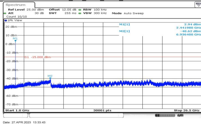
BLE 1M Ant1 2442 1000~26500
