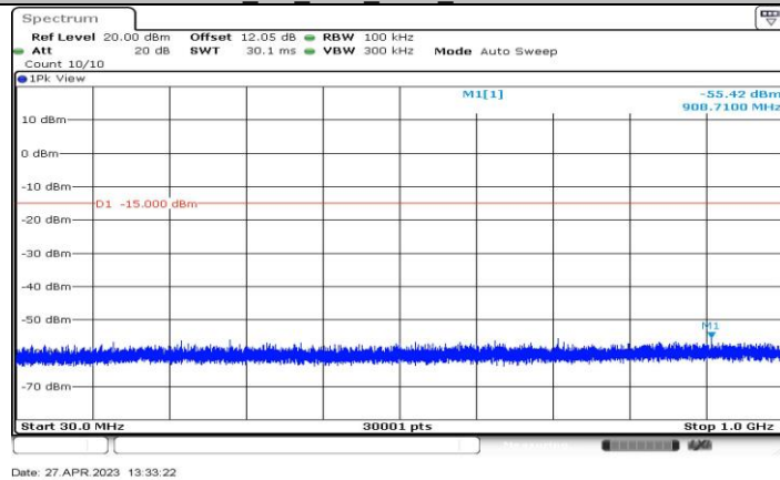
BLE 1M Ant1 2442 30~1000
