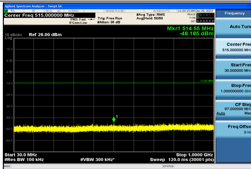
Band2-20MHz-16QAM-19100-1RB#0-30~1000MHz
