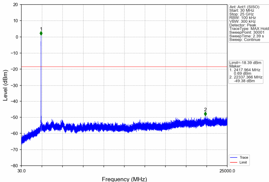
802.11n(HT20)_LCH_2412MHz_Ant1 (SISO)_NTNV
