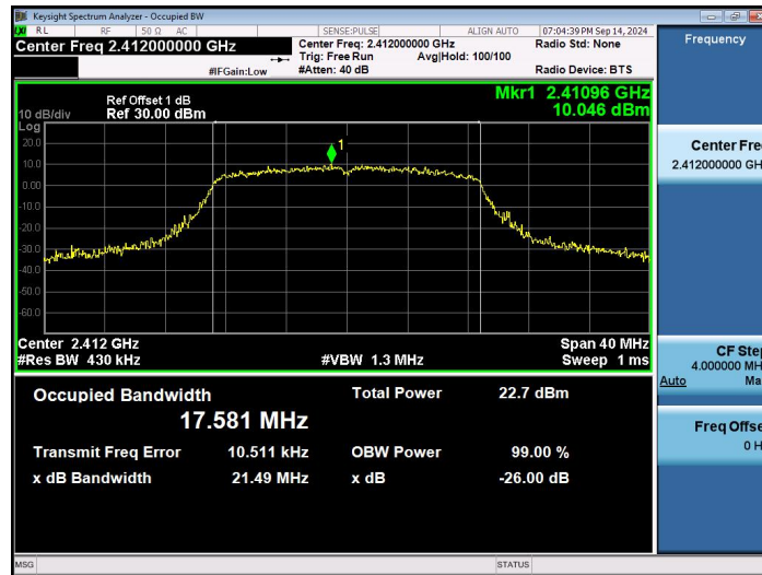
802.11n(HT20)SISO-Ant1-2412
