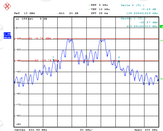
433.93MHz
