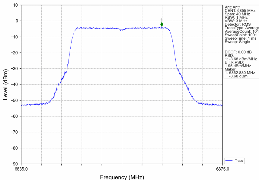
802.11ax(HEW20)_HCH_6855MHz_RU242_Left_Ant1_NTNV
