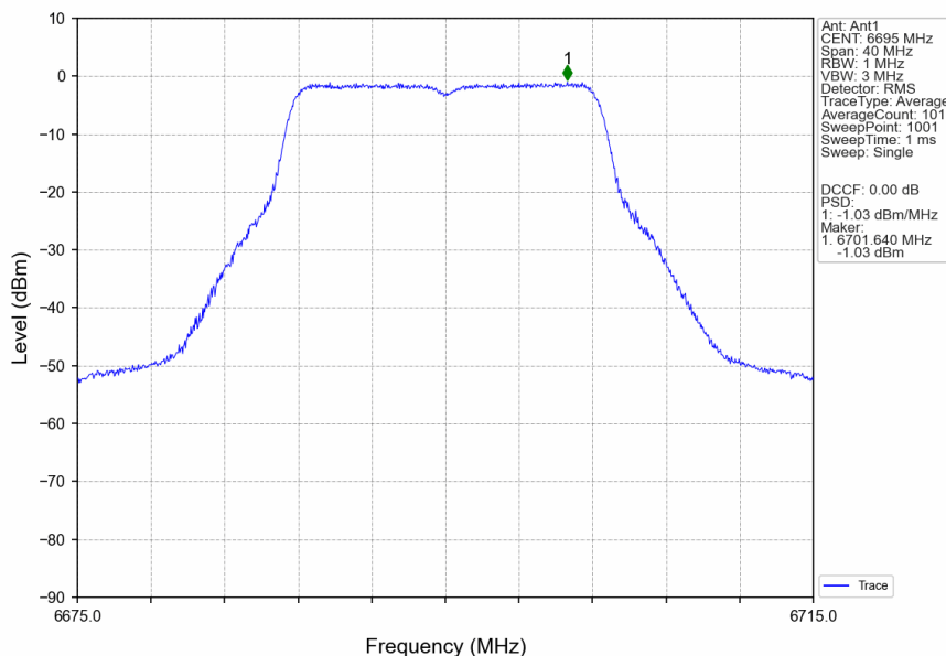
802.11a_MCH_6695MHz_Ant1_NTNV
