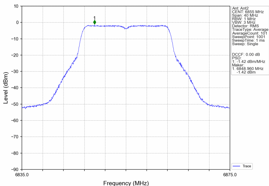
802.11a_HCH_6855MHz_Ant2_NTNV
