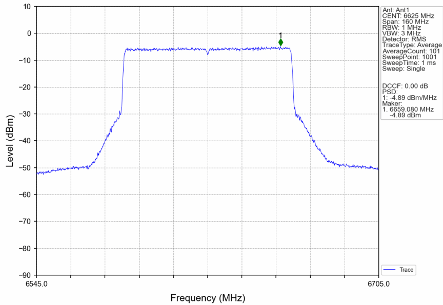
802.11ax(HEW80)_LCH_6625MHz_RU996_Left_Ant1_NTNV
