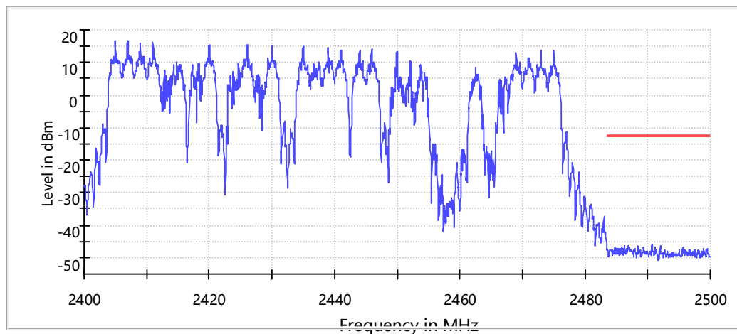
Band Edge
