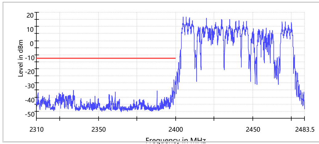
Band Edge
