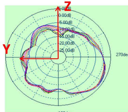
E1 (Phi=90)
