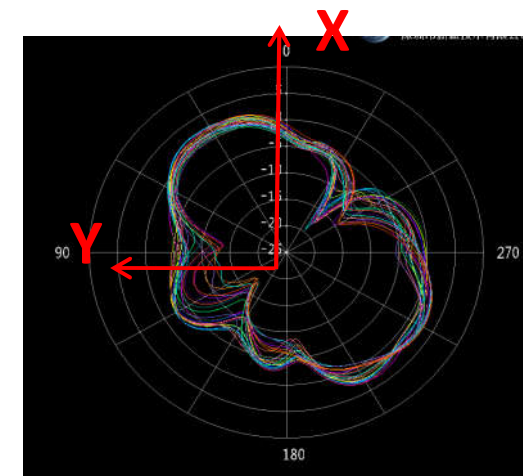
H ( \Theta=90 )
