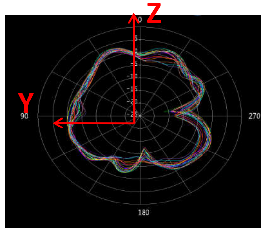
E1 ( \Phi=90 )
