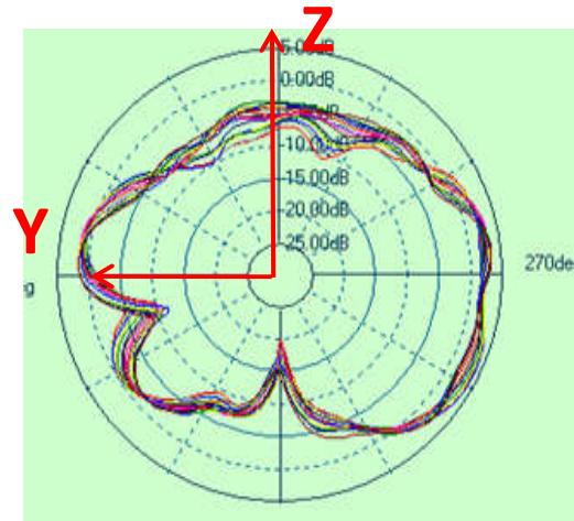
E1 (Phi=90)
