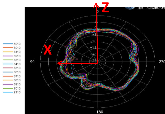
E1 ( \Phi=0 )
