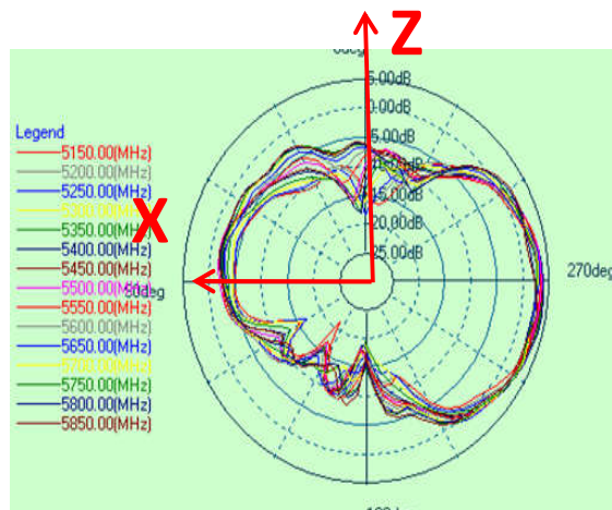
E1 (Phi=0)
