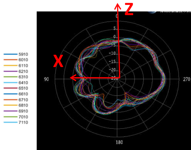
E1 ( \Phi=0 )
