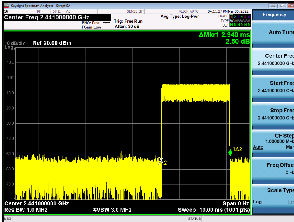
GFSK 2441MHz
