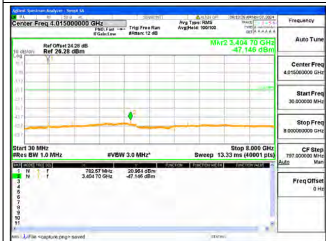
B13 / 5MHz / High CH / QPSK
