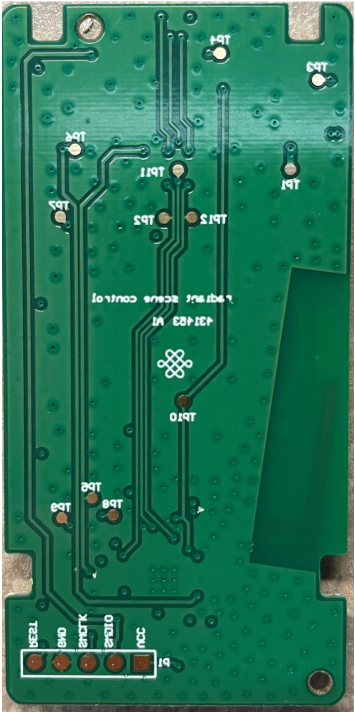
PCBA - BOT
