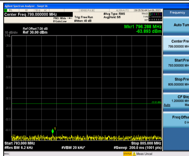
Band13-5MHz-16QAM-23230-1-0-Low-793-805--63.89-PASS
