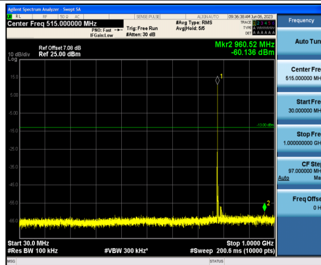
Band13-5MHz-16QAM-23255-1-0-Low-30-1000--60.14-PASS
