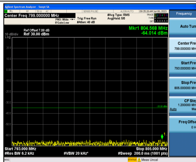
Band13-5MHz-QPSK-23230-1-0-Low-793-805--64.01-PASS
