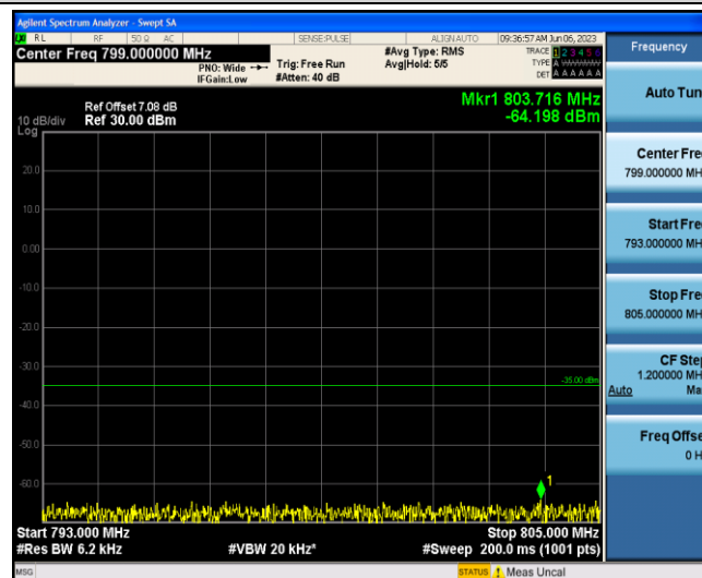
Band13-5MHz-16QAM-23255-1-0-Low-793-805--64.2-PASS
