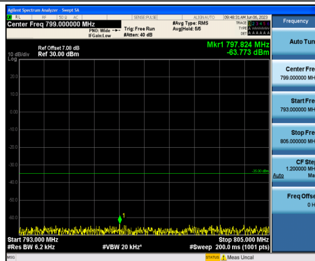
Band13-10MHz-16QAM-23230-1-0-Low-793-805--63.77-PASS
