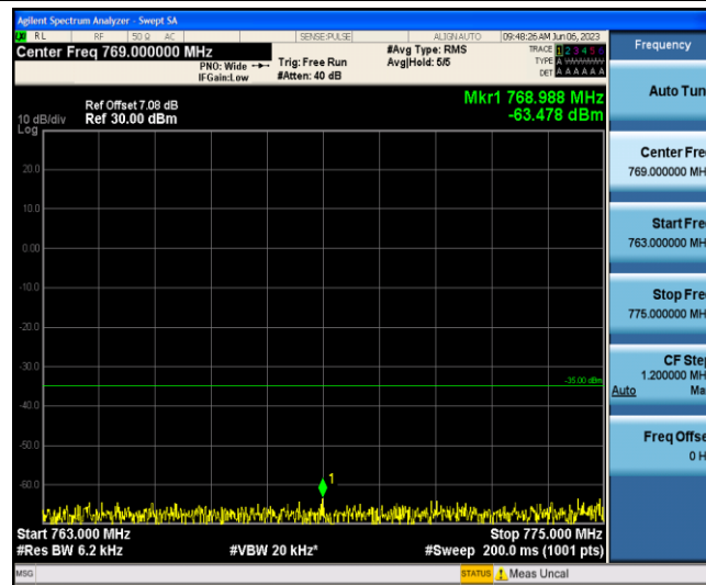
Band13-10MHz-16QAM-23230-1-0-Low-763-775--63.48-PASS
