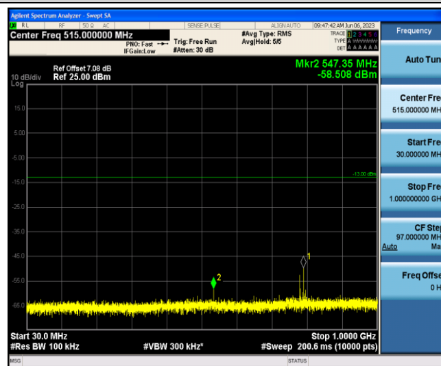
Band13-10MHz-QPSK-23230-1-0-Low-30-1000--58.51-PASS
