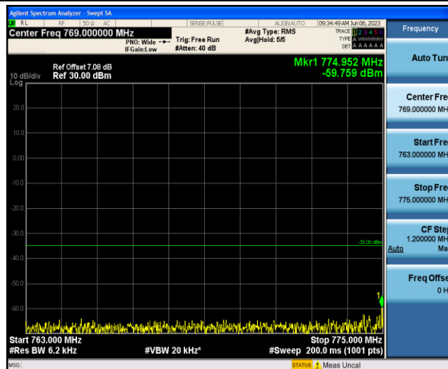
Band13-5MHz-16QAM-23205-1-0-Low-763-775--59.76-PASS
