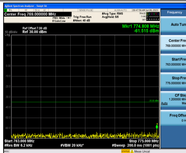
Band13-10MHz-QPSK-23230-1-0-Low-763-775--61.52-PASS
