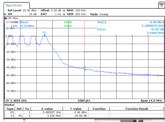
GFSK_Hopping_Upper
