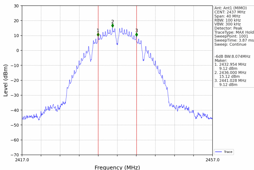
802.11b_MCH_2437MHz_Ant1 (MIMO)_NTNV
