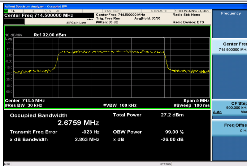
Band12-3MHz-QPSK-23165-15RB#0-2.6759
