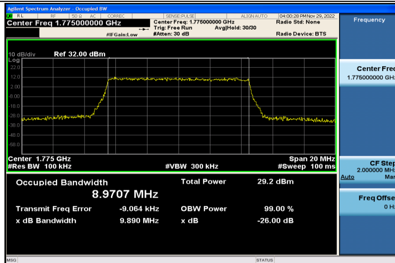
Band66-10MHz-QPSK-132622-50RB#0-8.9707
