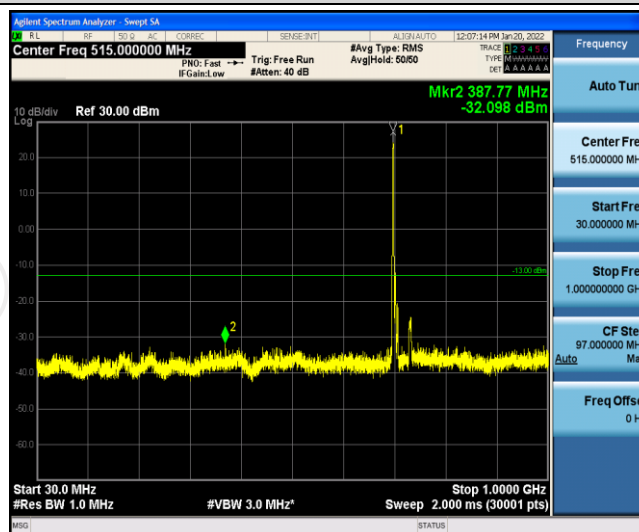
Band12-5MHz-QPSK-23095-1RB#0-Range4:1000~5000MHz
