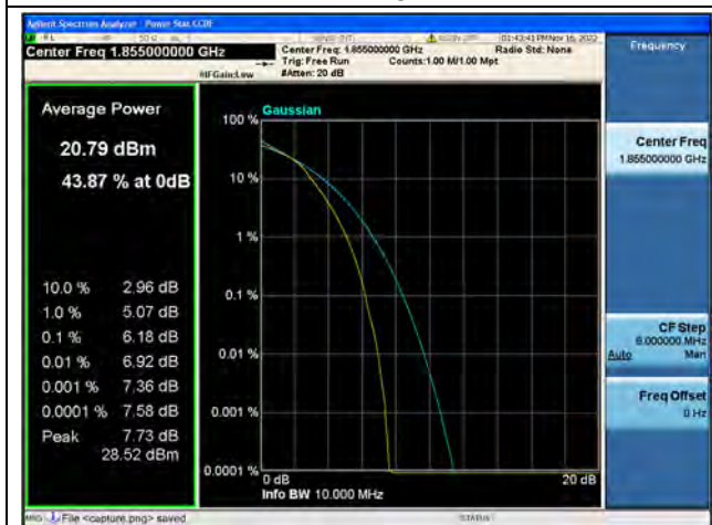
Band25 / 10MHz / Low CH / 16QAM
