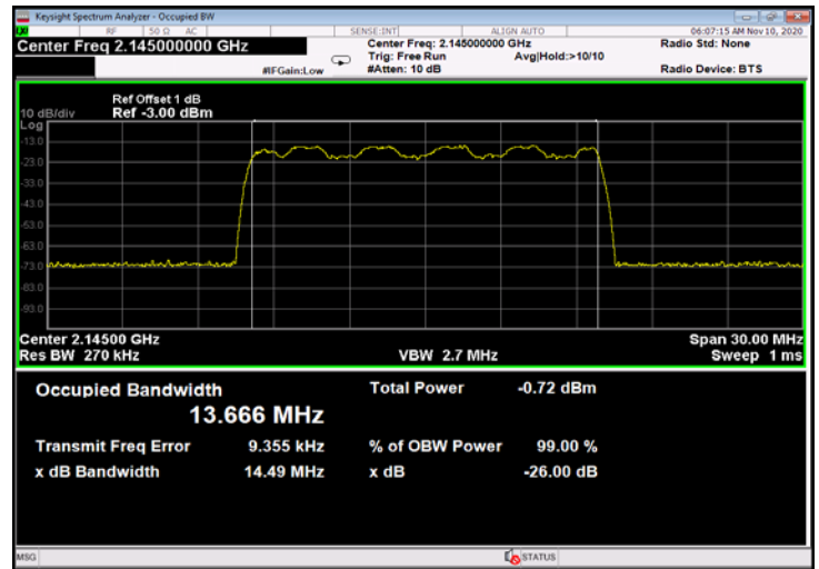
Figure 292: 16QAM 15MHz B.W.; 2145.0MHz, 30kHz - Input
