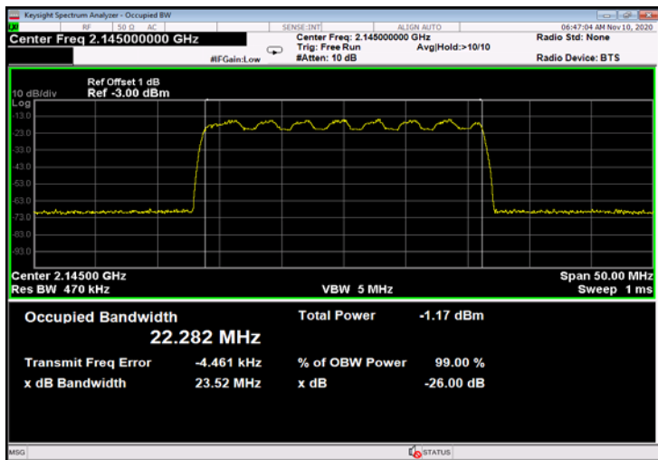
Figure 311: 16QAM 25MHz B.W.; 2145.0MHz, 60kHz - Input
