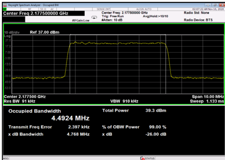
Figure 343: 64QAM 5MHz B.W.; 2177.5MHz, 15kHz - Input
