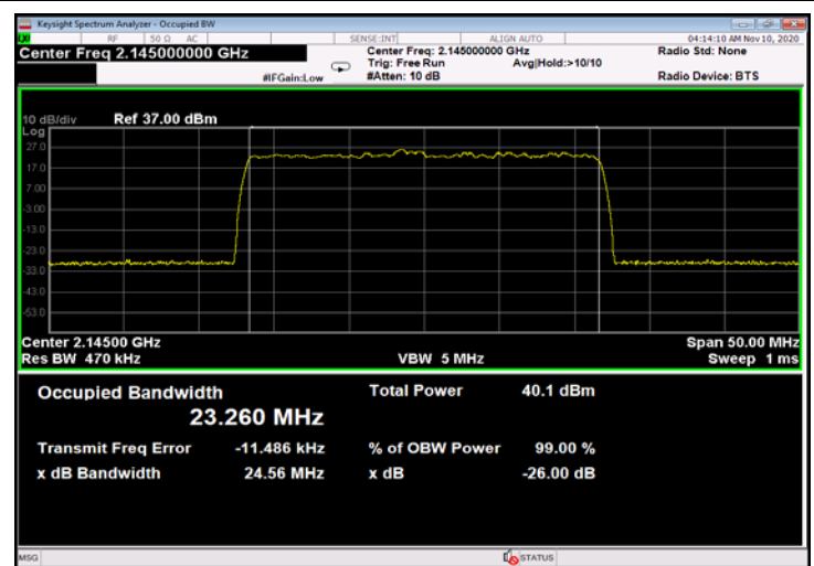
Figure 376: 64QAM 25MHz B.W.; 2145.0MHz, 30kHz - Input
