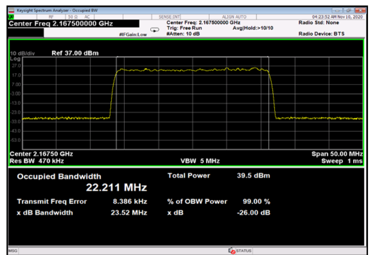
Figure 380: 64QAM 25MHz B.W.; 2167.5MHz, 60kHz - Input
