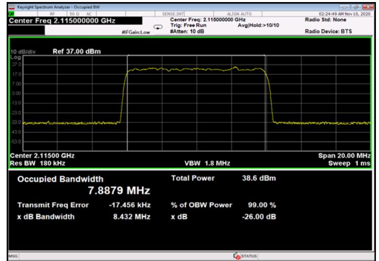
Figure 346: 64QAM 10MHz B.W.; 2115.0MHz, 30kHz - Input
