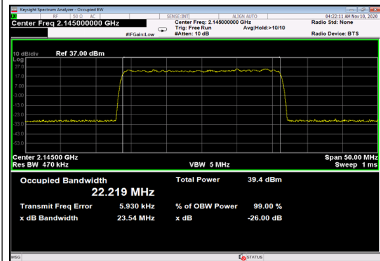
Figure 377: 64QAM 25MHz B.W.; 2145.0MHz, 60kHz - Input
