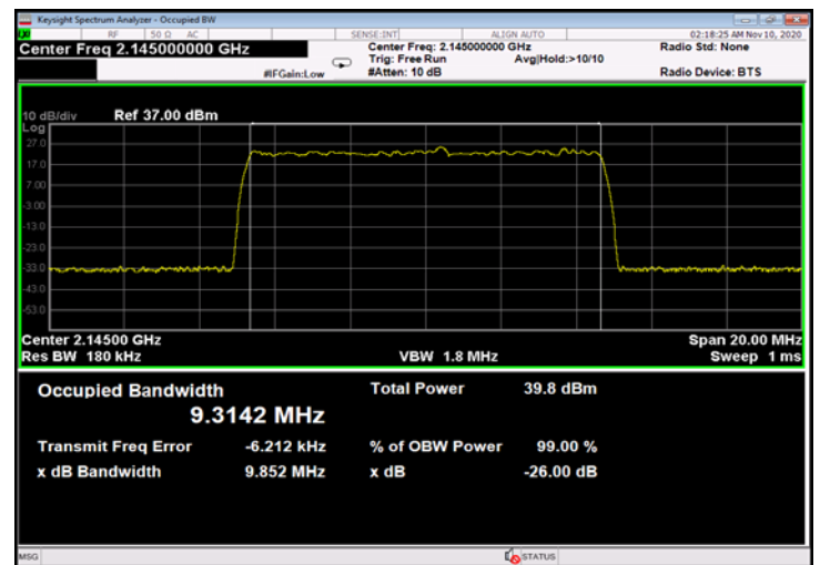
Figure 348: 64QAM 10MHz B.W.; 2145.0MHz, 15kHz - Input
