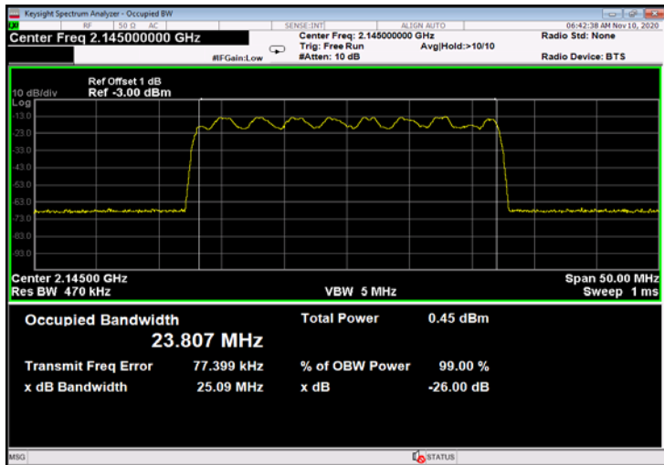
Figure 309: 16QAM 25MHz B.W.; 2145.0MHz, 15kHz - Input
