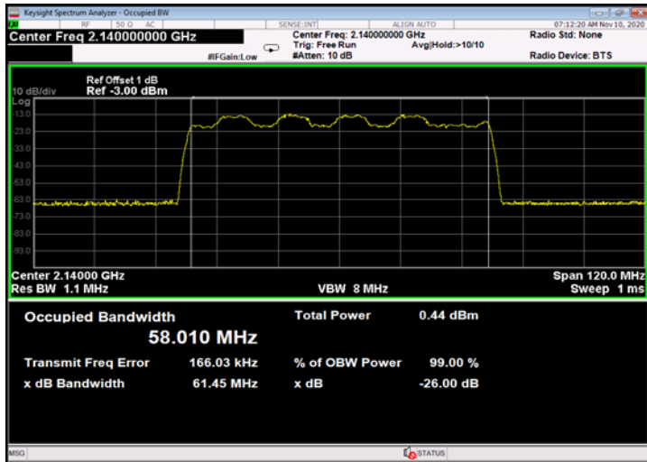
Figure 333: 16QAM 60MHz B.W.; 2140.0MHz, 30kHz - Input
