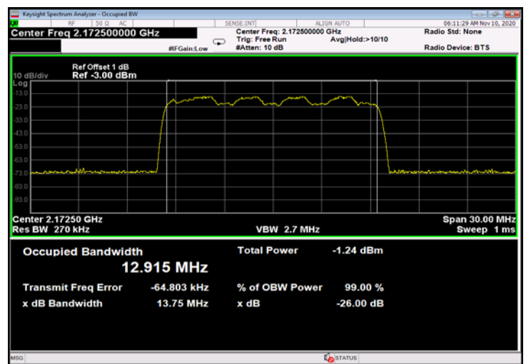
Figure 296: 16QAM 15MHz B.W.; 2172.5MHz, 60kHz - Input
