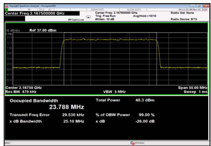
Figure 378: 64QAM 25MHz B.W.; 2167.5MHz, 15kHz - Input
