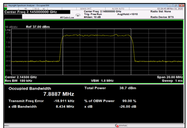
Figure 350: 64QAM 10MHz B.W.; 2145.0MHz, 60kHz - Input
