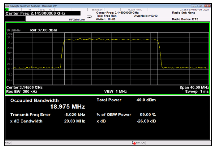
Figure 366: 64QAM 20MHz B.W.; 2145.0MHz, 15kHz - Input
