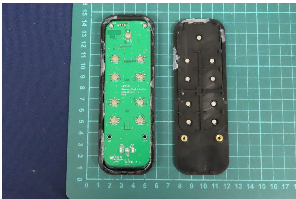
(57) EUT Photo
