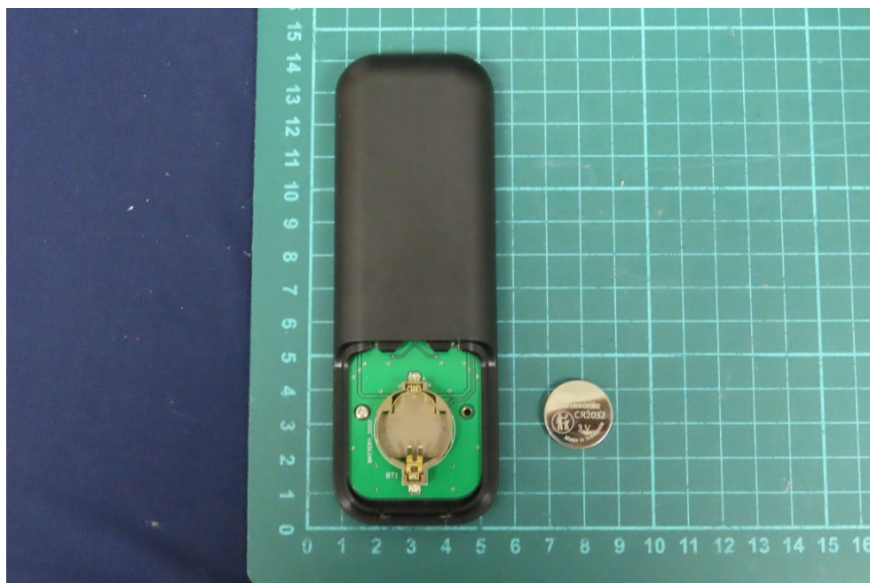
(53) EUT Photo
