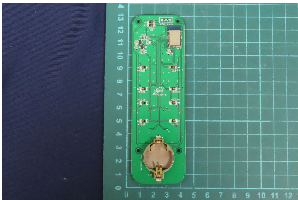
(61) EUT Photo
