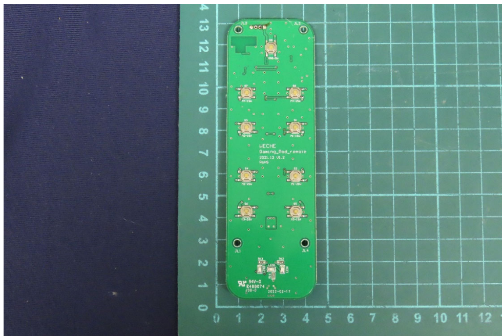
(60) EUT Photo
