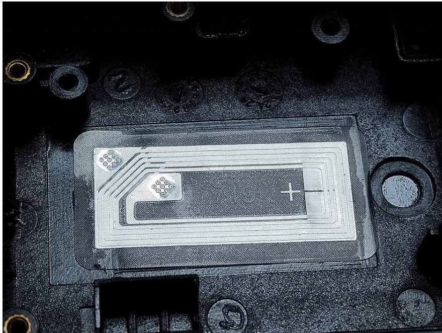
NFC Antenna
