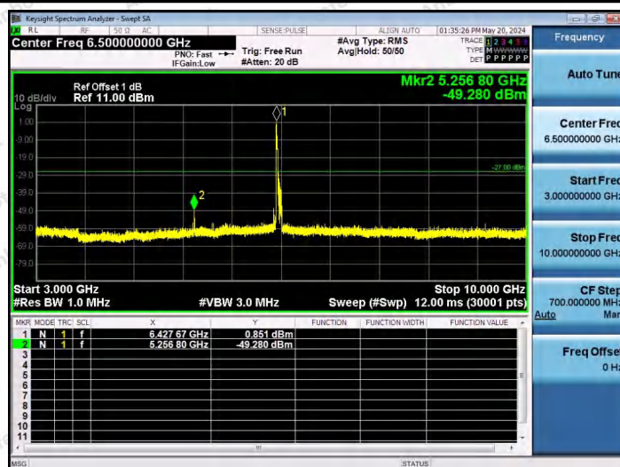
11AX80SISO-Ant1-6465-52Tone-RU37-3000~10000-PASS
