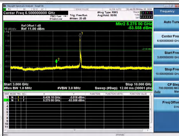
11AX80SISO-Ant1-6465-242Tone-RU61-3000~10000-PASS
