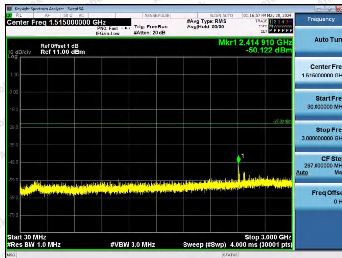
11AX80SISO-Ant1-6385-242Tone-RU64-30~3000-PASS
