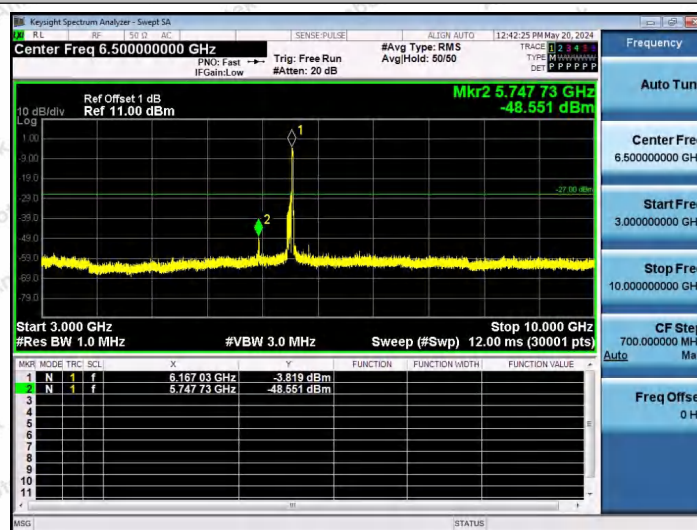
11AX80SISO-Ant1-6145-242Tone-RU64-3000~10000-PASS
