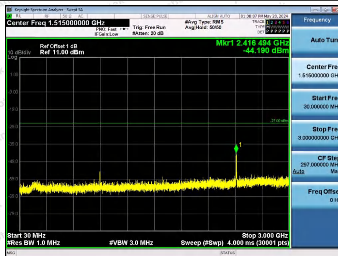
11AX80SISO-Ant1-6385-106Tone-RU60-30~3000-PASS
