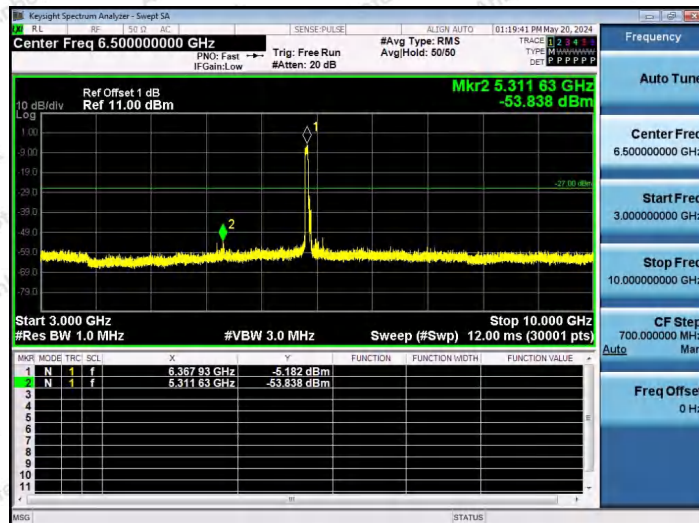
11AX80SISO-Ant1-6385-484Tone-RU65-3000~10000-PASS
