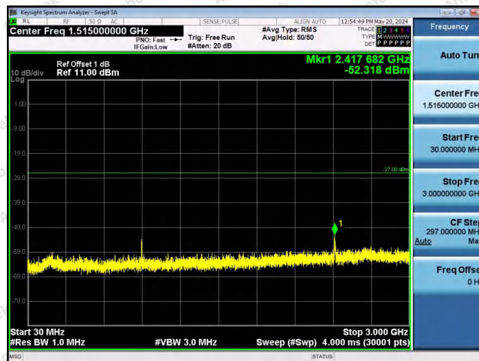
11AX80SISO-Ant1-6385-26Tone-RU36-30~3000-PASS
