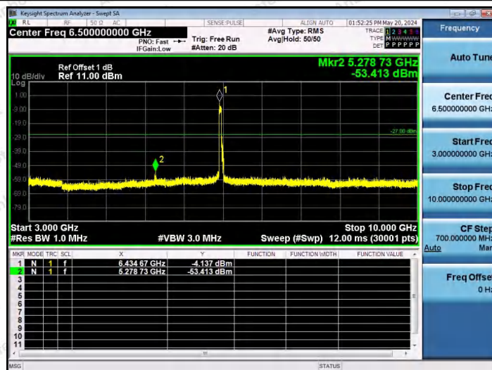
11AX80SISO-Ant1-6465-484Tone-RU65-3000~10000-PASS
