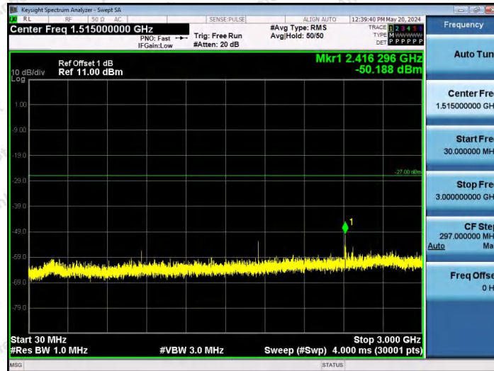
11AX80SISO-Ant1-6145-242Tone-RU61-30~3000-PASS
