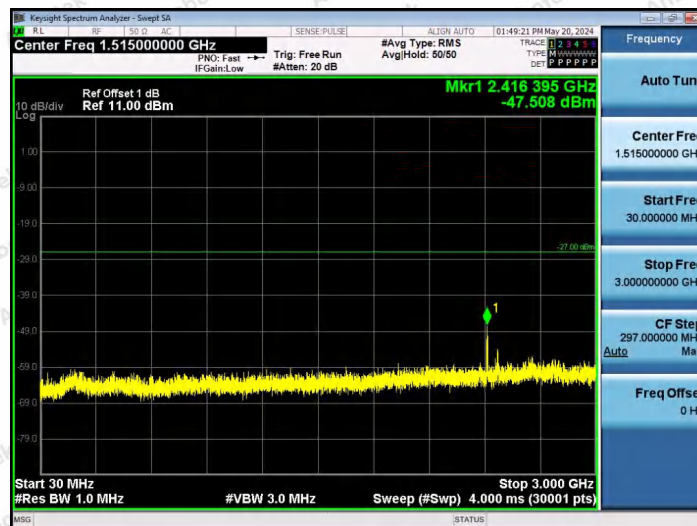
11AX80SISO-Ant1-6465-242Tone-RU64-30~3000-PASS
