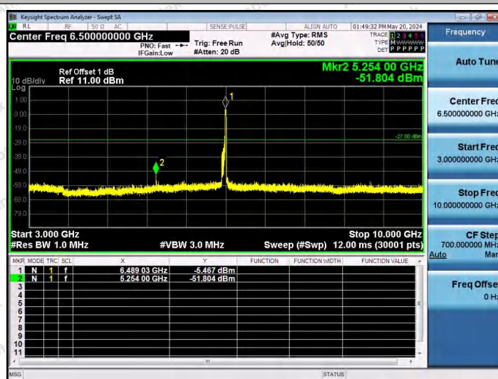
11AX80SISO-Ant1-6465-242Tone-RU64-3000~10000-PASS
