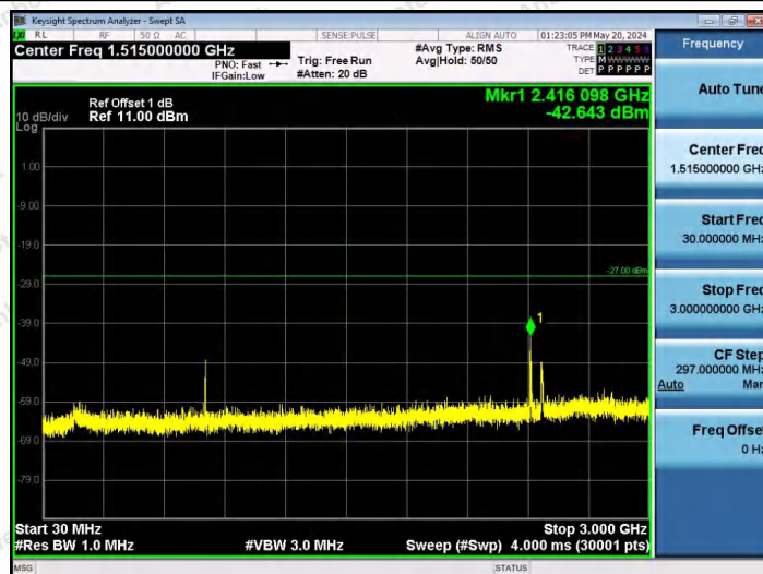
11AX80SISO-Ant1-6385-484Tone-RU66-30~3000-PASS
