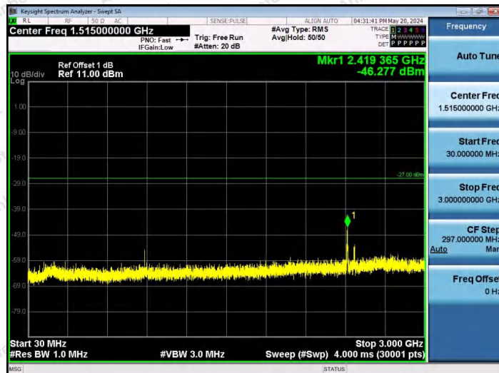
11AX80SISO-Ant1-6705-484Tone-RU66-30~3000-PASS
