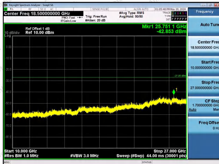
11AX80SISO-Ant1-6385-106Tone-RU53-10000~40000-PASS
