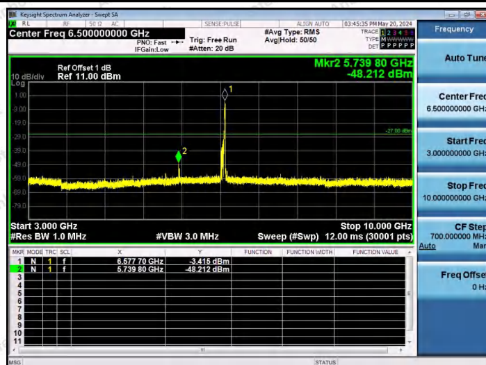
11AX80SISO-Ant1-6545-106Tone-RU60-3000~10000-PASS
