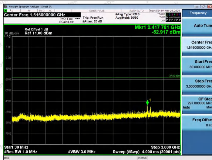
11AX80SISO-Ant1-6545-106Tone-RU60-30~3000-PASS
