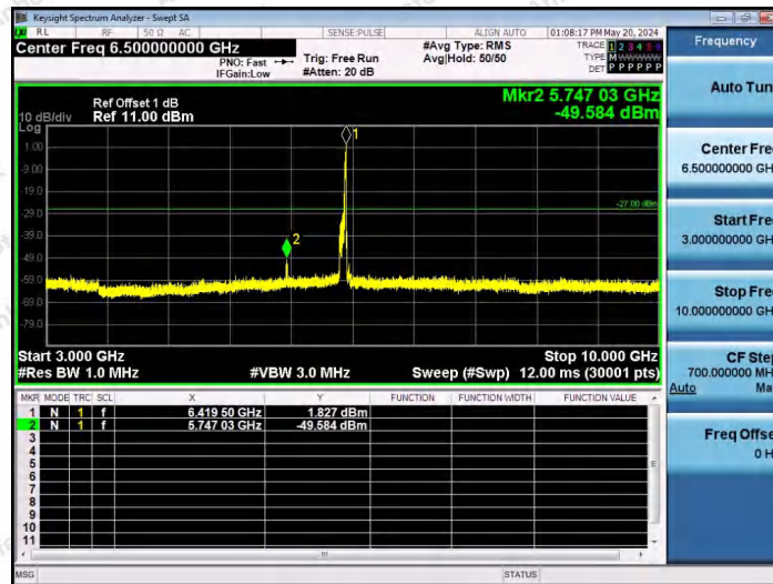
11AX80SISO-Ant1-6385-106Tone-RU60-3000~10000-PASS
