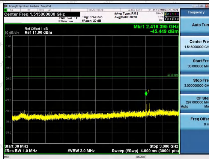
11AX80SISO-Ant1-6465-52Tone-RU37-30~3000-PASS
