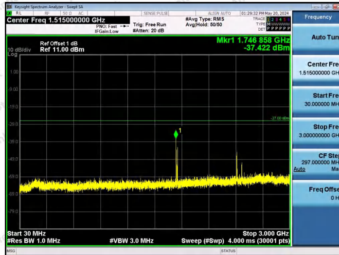
11AX80SISO-Ant1-6465-26Tone-RU0-30~3000-PASS
