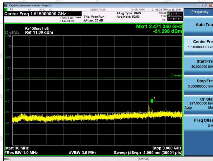
11AX80SISO-Ant1-6385-106Tone-RU53-30~3000-PASS
