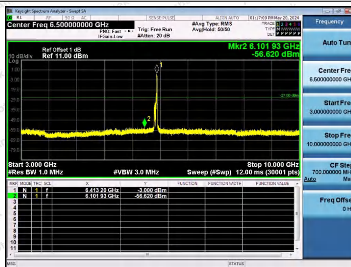
11AX80SISO-Ant1-6385-242Tone-RU64-3000~10000-PASS
