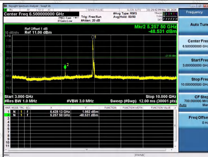
11AX80SISO-Ant1-6465-26Tone-RU0-3000~10000-PASS
