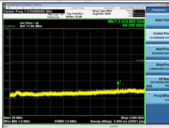
11AX80SISO-Ant1-6465-484Tone-RU65-30~3000-PASS
