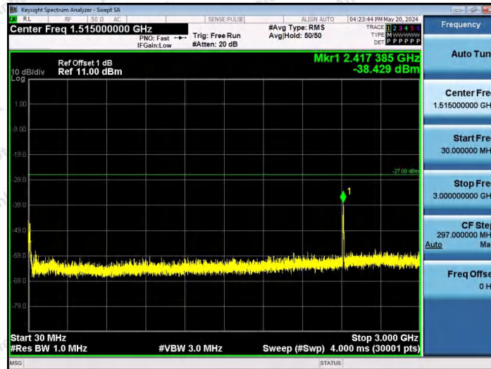
11AX80SISO-Ant1-6705-242Tone-RU61-30~3000-PASS
