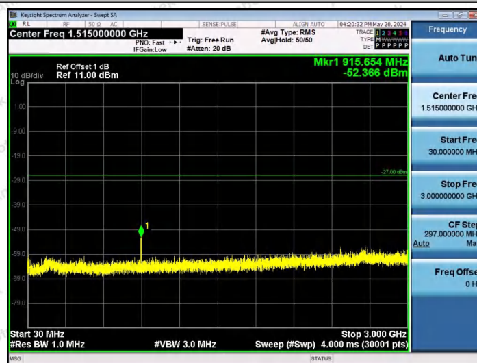
11AX80SISO-Ant1-6705-106Tone-RU60-30~3000-PASS
