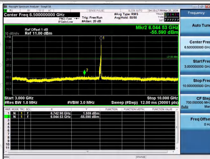
11AX80SISO-Ant1-6705-26Tone-RU36-3000~10000-PASS
