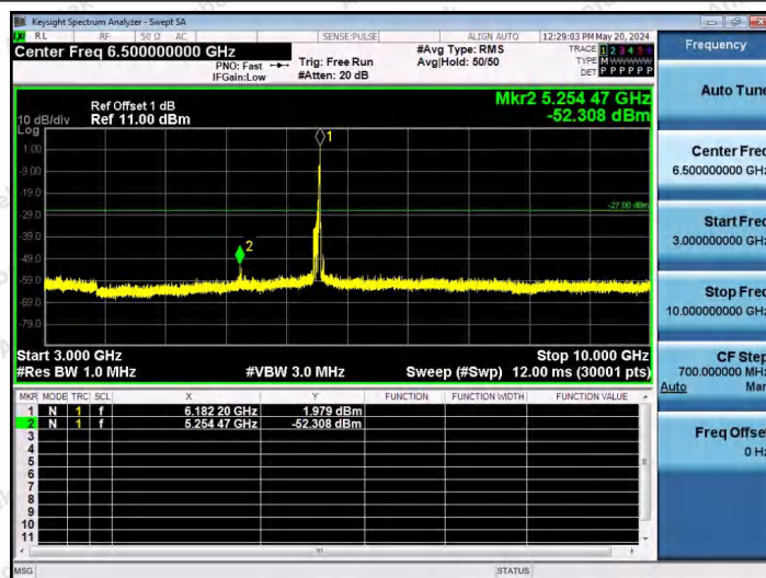
11AX80SISO-Ant1-6145-52Tone-RU52-3000~10000-PASS
