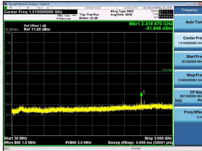
11AX80SISO-Ant1-6545-26Tone-RU0-30~3000-PASS
