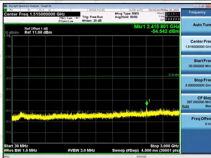
11AX80SISO-Ant1-6545-106Tone-RU53-30~3000-PASS
