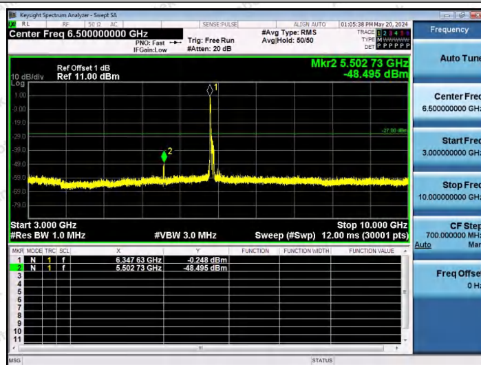
11AX80SISO-Ant1-6385-106Tone-RU53-3000~10000-PASS
