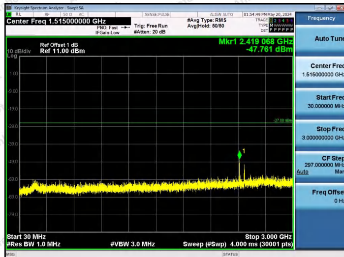
11AX80SISO-Ant1-6465-484Tone-RU66-30~3000-PASS
