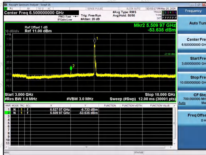
11AX80SISO-Ant1-6545-484Tone-RU65-3000~10000-PASS
