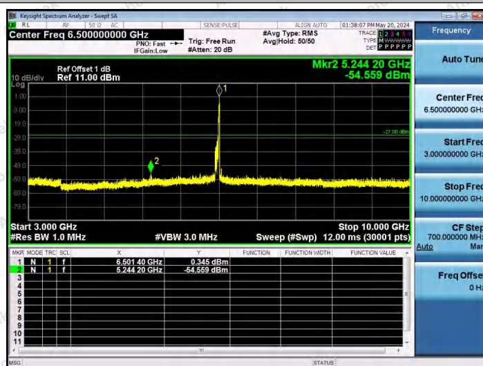
11AX80SISO-Ant1-6465-52Tone-RU52-3000~10000-PASS
