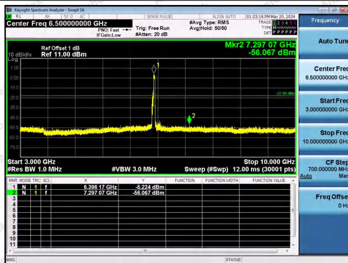
11AX80SISO-Ant1-6385-484Tone-RU66-3000~10000-PASS
