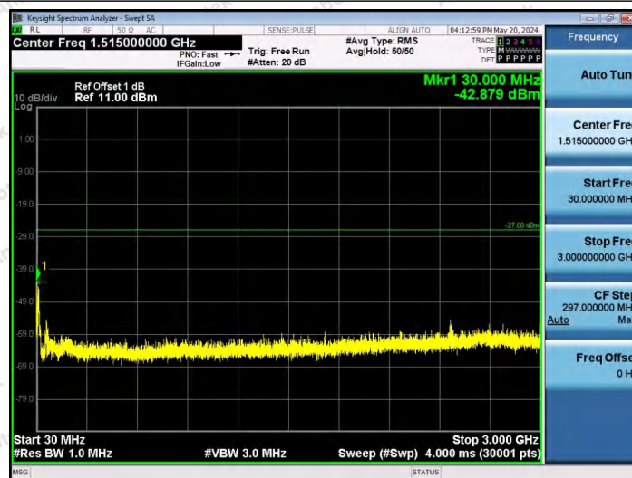
11AX80SISO-Ant1-6705-52Tone-RU37-30~3000-PASS
