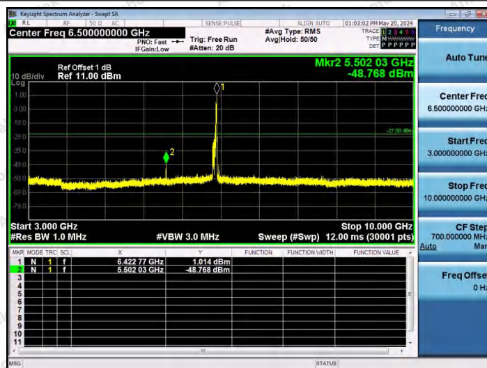
11AX80SISO-Ant1-6385-52Tone-RU52-3000~10000-PASS
