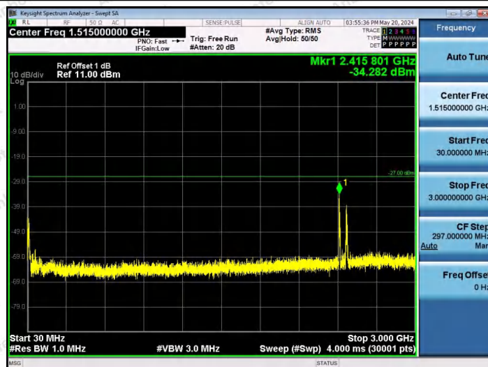
11AX80SISO-Ant1-6545-484Tone-RU66-30~3000-PASS
