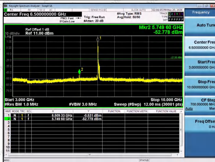
11AX80SISO-Ant1-6545-52Tone-RU37-3000~10000-PASS
