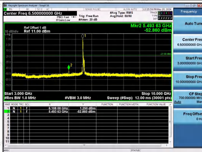
11AX80SISO-Ant1-6145-52Tone-RU37-3000~10000-PASS
