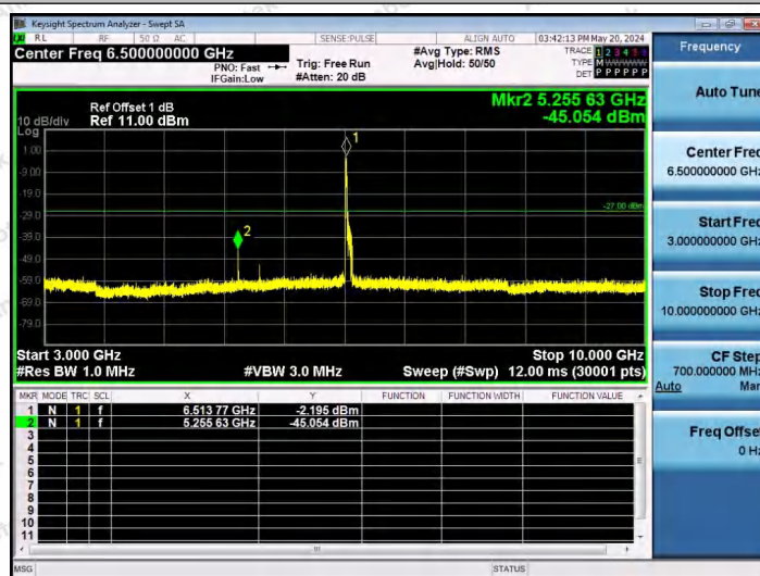
11AX80SISO-Ant1-6545-106Tone-RU53-3000~10000-PASS
