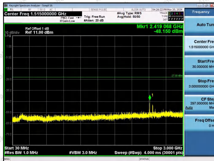
11AX80SISO-Ant1-6705-242Tone-RU64-30~3000-PASS
