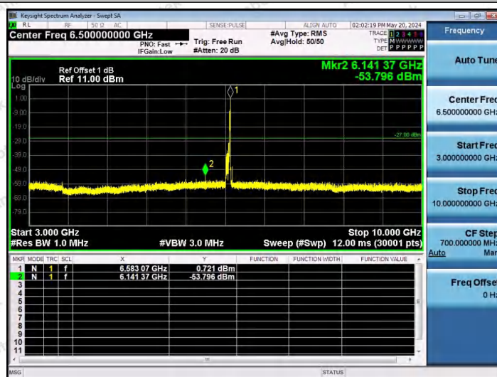
11AX80SISO-Ant1-6545-26Tone-RU36-3000~10000-PASS
