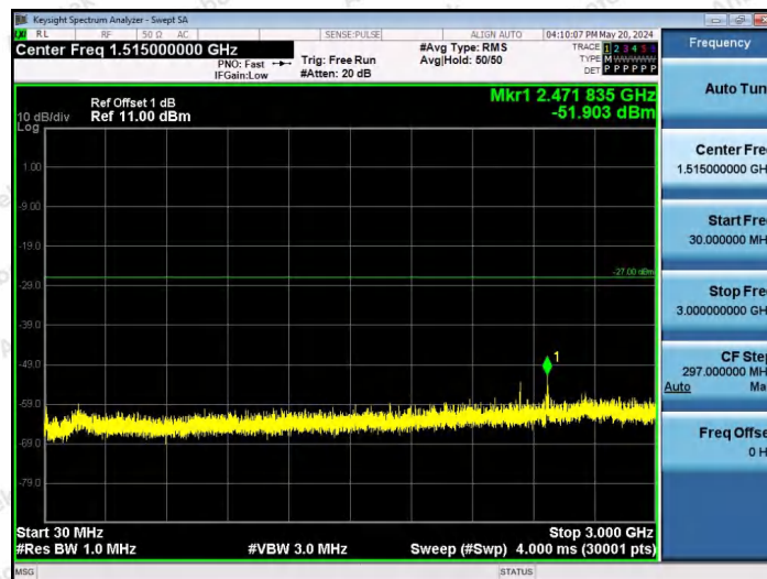
11AX80SISO-Ant1-6705-26Tone-RU36-30~3000-PASS
