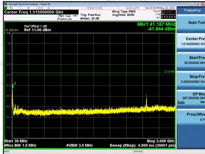
11AX80SISO-Ant1-6705-52Tone-RU52-30~3000-PASS
