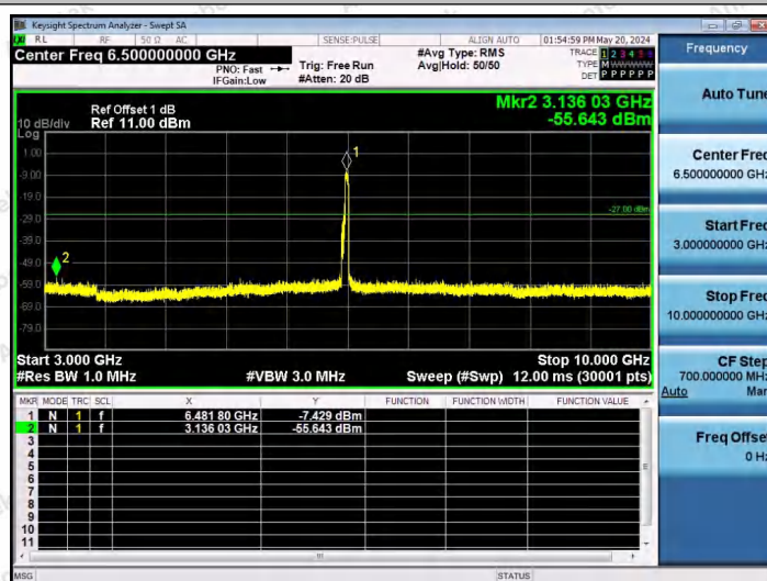
11AX80SISO-Ant1-6465-484Tone-RU66-3000~10000-PASS
