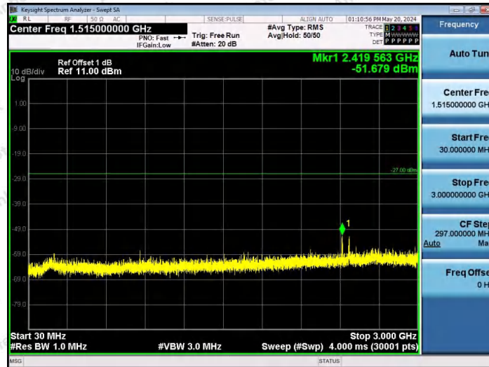
11AX80SISO-Ant1-6385-242Tone-RU61-30~3000-PASS
