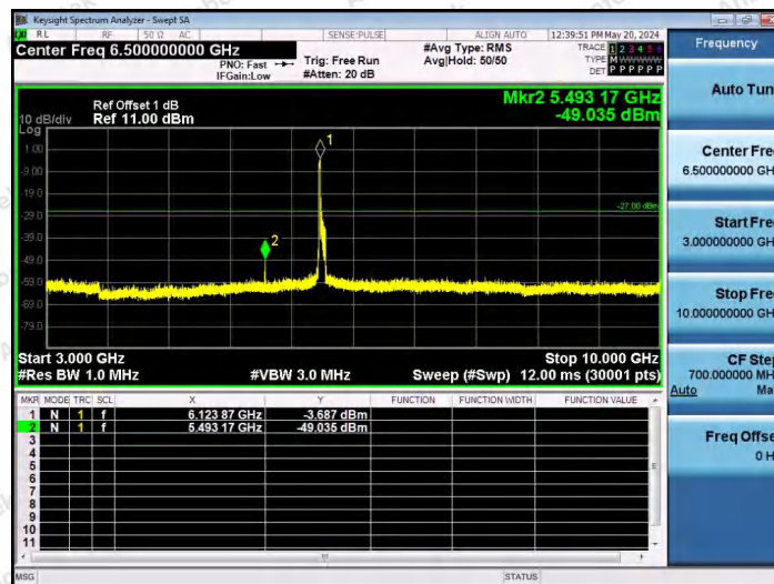
11AX80SISO-Ant1-6145-242Tone-RU61-3000~10000-PASS
