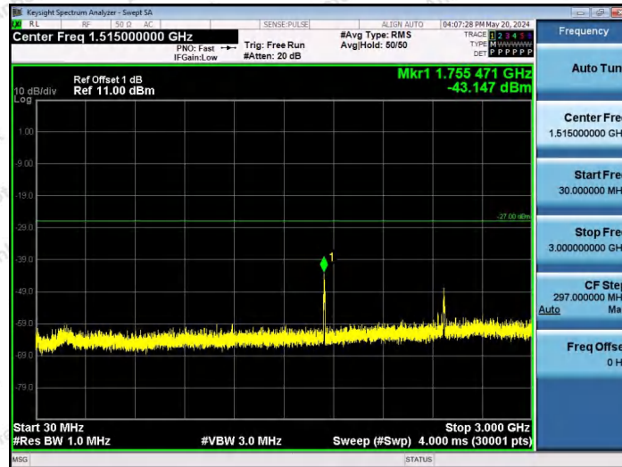
11AX80SISO-Ant1-6705-26Tone-RU0-30~3000-PASS
