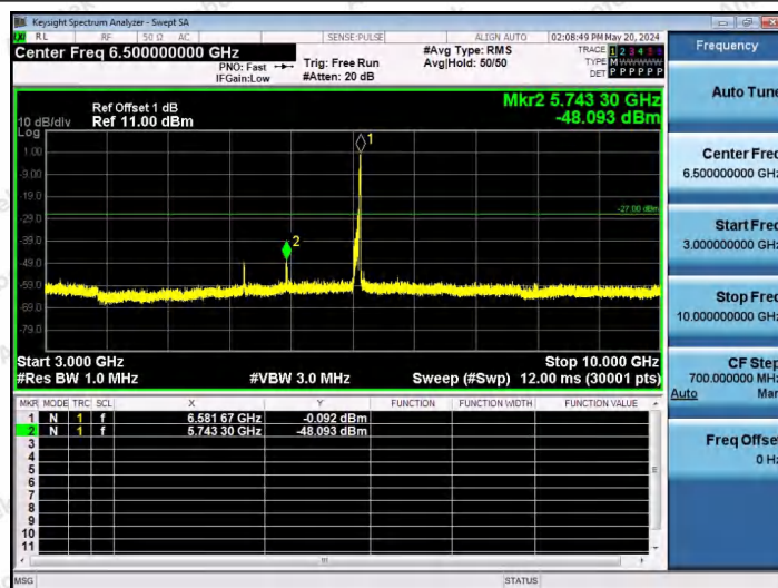
11AX80SISO-Ant1-6545-52Tone-RU52-3000~10000-PASS
