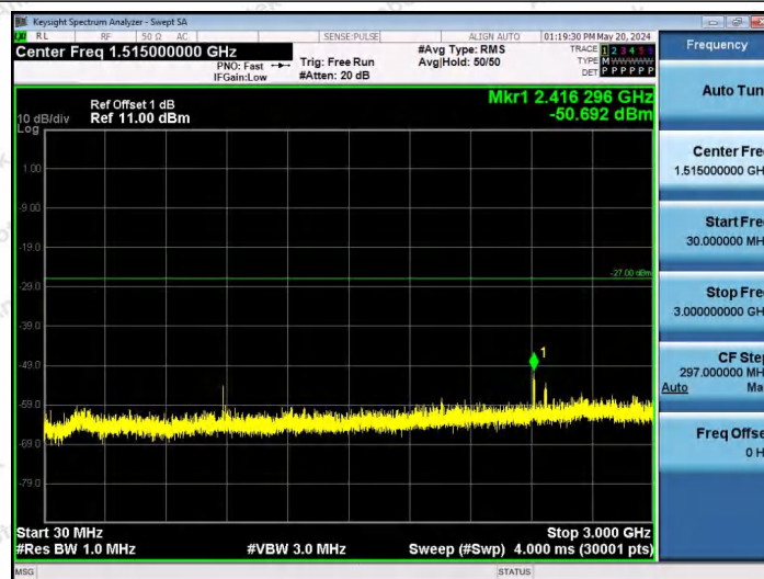
11AX80SISO-Ant1-6385-484Tone-RU65-30~3000-PASS
