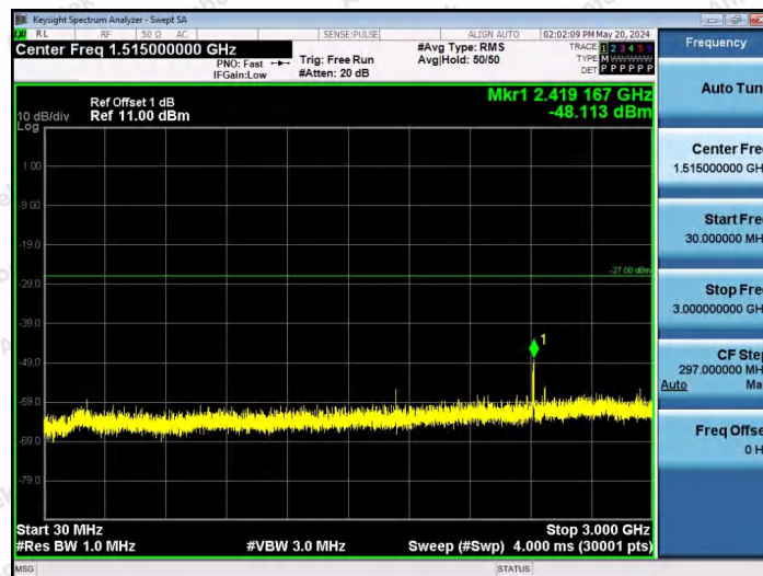
11AX80SISO-Ant1-6545-26Tone-RU36-30~3000-PASS
