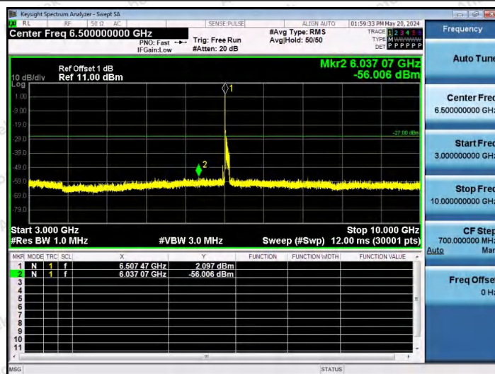
11AX80SISO-Ant1-6545-26Tone-RU0-3000~10000-PASS
