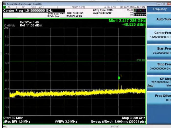
11AX80SISO-Ant1-6545-52Tone-RU52-30~3000-PASS
