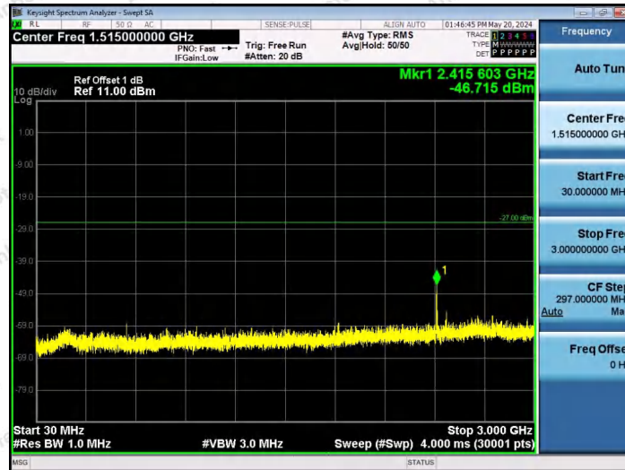
11AX80SISO-Ant1-6465-242Tone-RU61-30~3000-PASS
