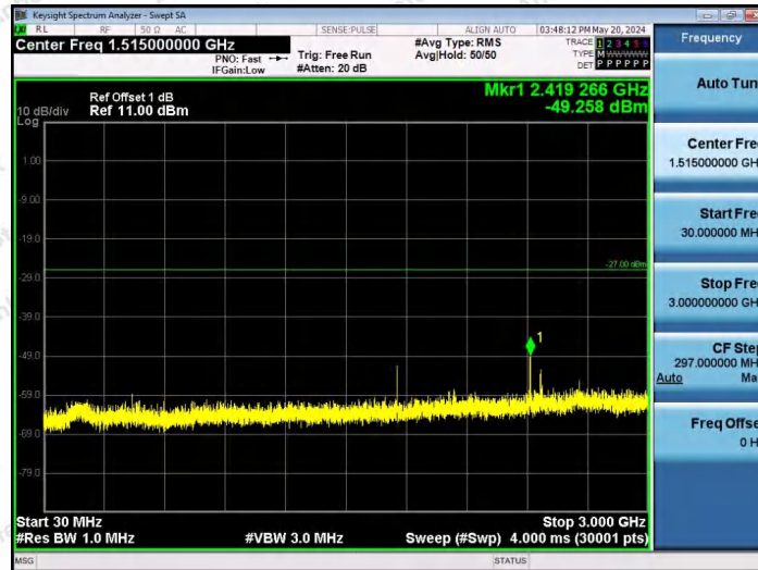
11AX80SISO-Ant1-6545-242Tone-RU61-30~3000-PASS
