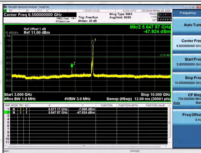
11AX80SISO-Ant1-6545-242Tone-RU64-3000~10000-PASS
