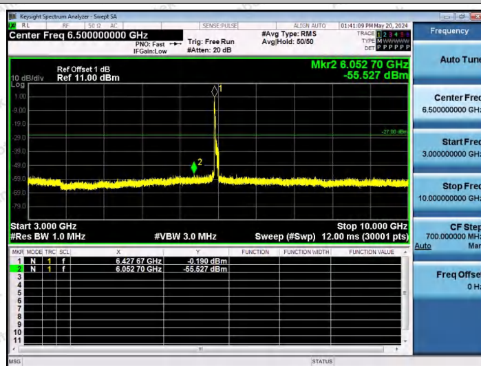
11AX80SISO-Ant1-6465-106Tone-RU53-3000~10000-PASS
