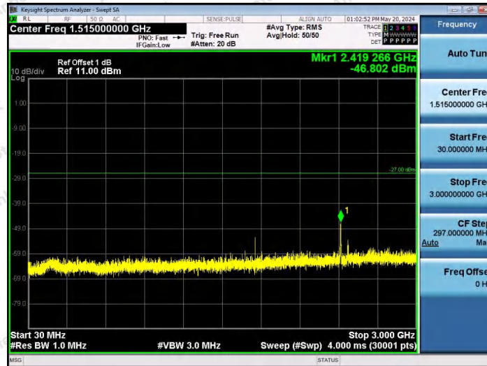
11AX80SISO-Ant1-6385-52Tone-RU52-30~3000-PASS
