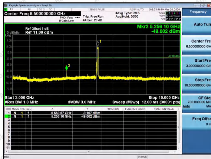
11AX80SISO-Ant1-6545-484Tone-RU66-3000~10000-PASS
