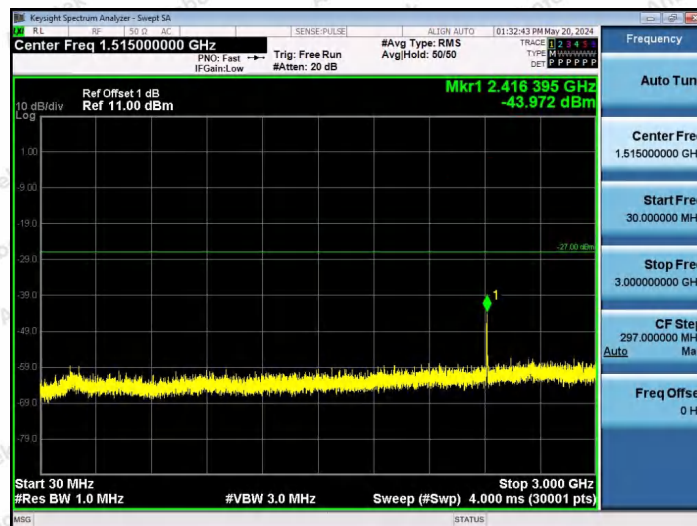
11AX80SISO-Ant1-6465-26Tone-RU36-30~3000-PASS
