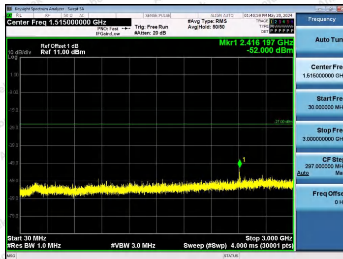
11AX80SISO-Ant1-6465-106Tone-RU53-30~3000-PASS
