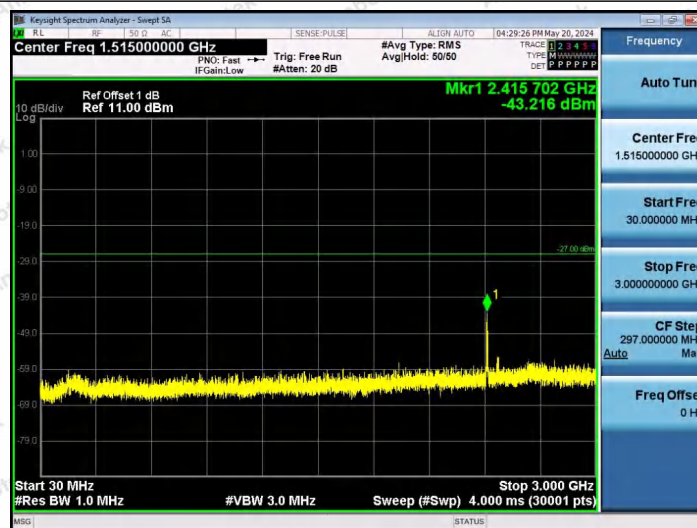
11AX80SISO-Ant1-6705-484Tone-RU65-30~3000-PASS
