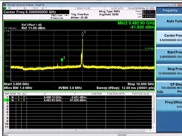
11AX80SISO-Ant1-6465-106Tone-RU60-3000~10000-PASS
