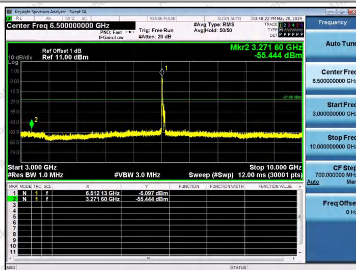
11AX80SISO-Ant1-6545-242Tone-RU61-3000~10000-PASS
