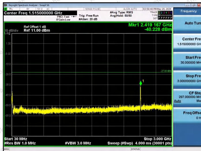
11AX80SISO-Ant1-6545-242Tone-RU64-30~3000-PASS
