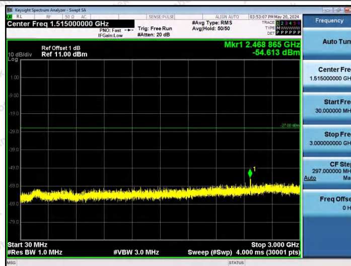
11AX80SISO-Ant1-6545-484Tone-RU65-30~3000-PASS
