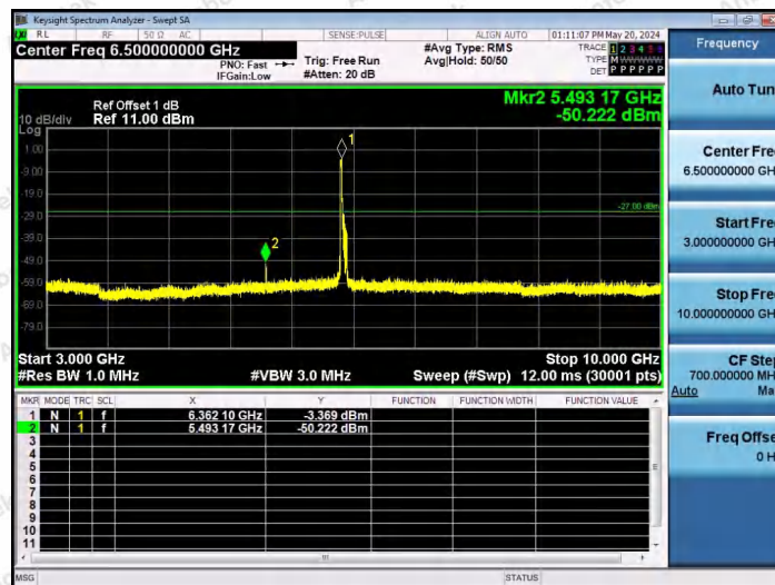
11AX80SISO-Ant1-6385-242Tone-RU61-3000~10000-PASS
