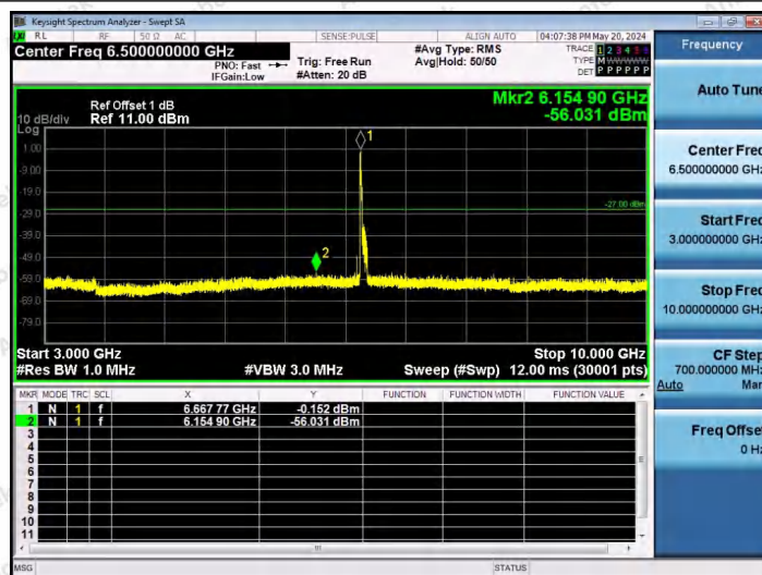
11AX80SISO-Ant1-6705-26Tone-RU0-3000~10000-PASS
