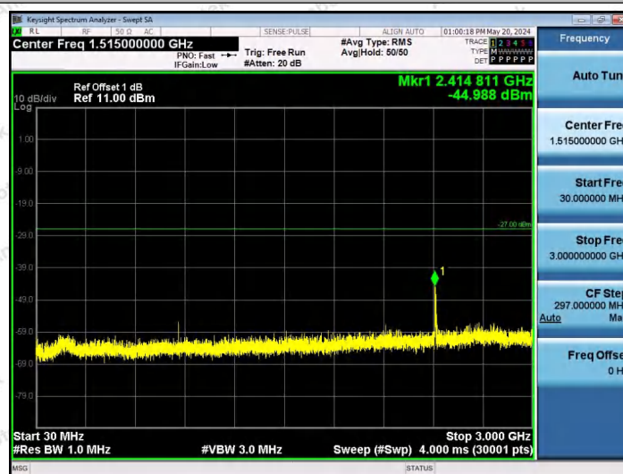
11AX80SISO-Ant1-6385-52Tone-RU37-30~3000-PASS
