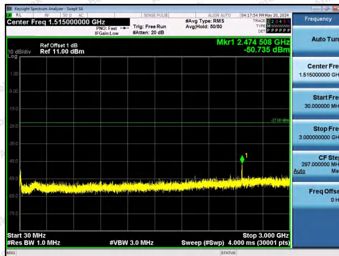
11AX80SISO-Ant1-6705-106Tone-RU53-30~3000-PASS
