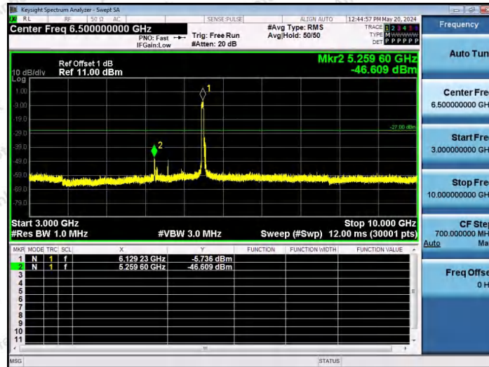
11AX80SISO-Ant1-6145-484Tone-RU65-3000~10000-PASS
