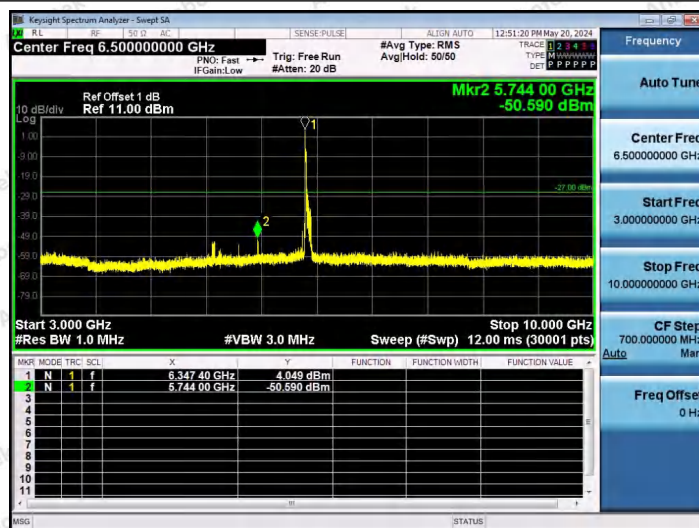
11AX80SISO-Ant1-6385-26Tone-RU0-3000~10000-PASS
