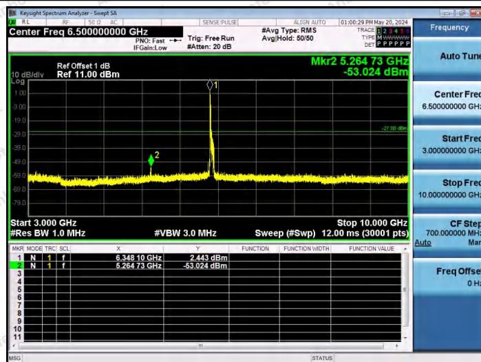
11AX80SISO-Ant1-6385-52Tone-RU37-3000~10000-PASS
