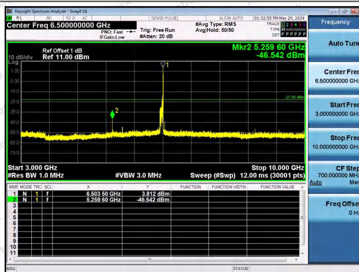
11AX80SISO-Ant1-6465-26Tone-RU36-3000~10000-PASS
