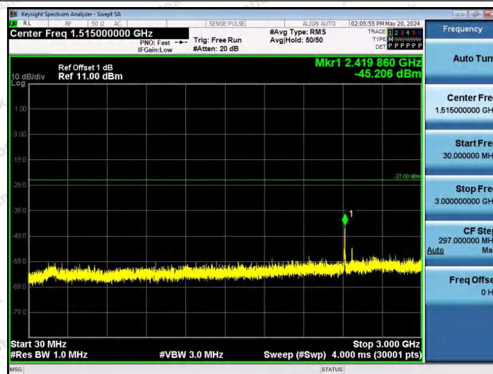
11AX80SISO-Ant1-6545-52Tone-RU37-30~3000-PASS
