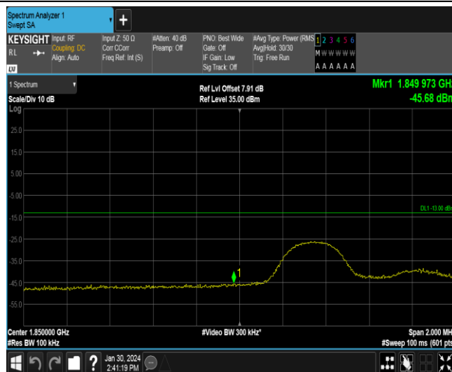
Band2-5MHz-QPSK-18625-1RB#24
