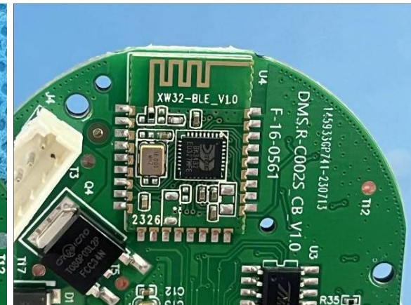
RF Module
