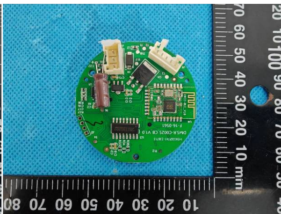
RF Module
