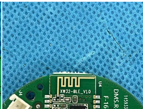
Antenna
