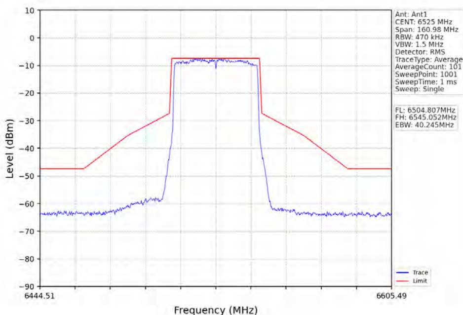
802.11ax(HEW80)_HCH_6545MHz_RU484_Left_Ant1_NTNV
