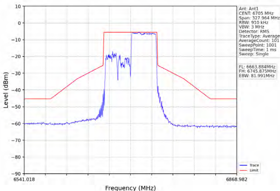
802.11ax(HEW80)_MCH_6705MHz_RU996_Left_Ant1_NTNV
