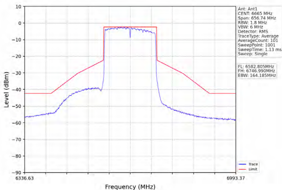
802.11ax(HEW160)_MCH_6665MHz_2xRU996_Left_Ant1_NTNV
