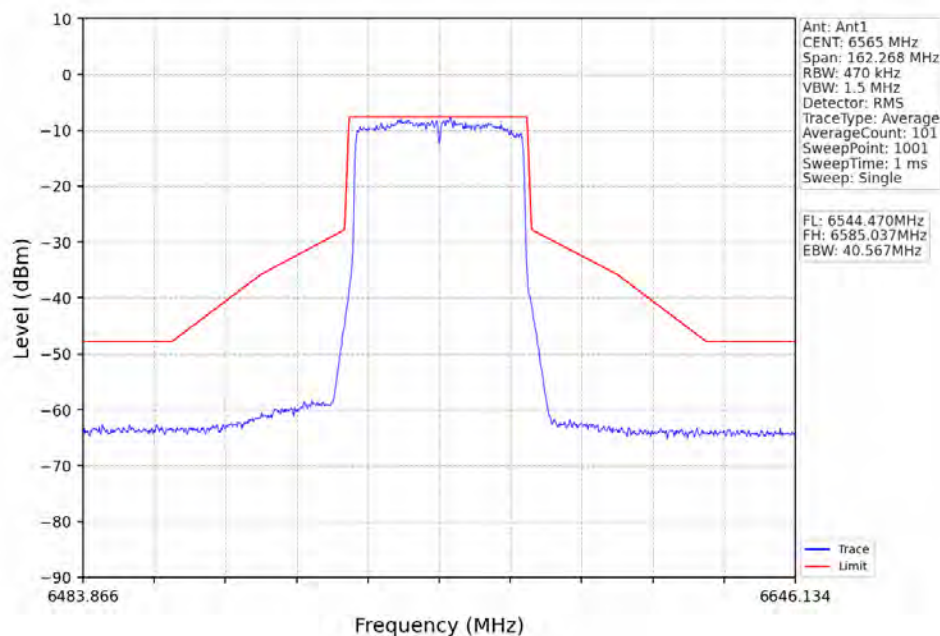
802.11ax(HEW40)_LCH_6565MHz_RU484_Left_Ant1_NTNV
