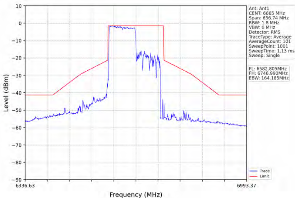
802.11ax(HEW160)_MCH_6665MHz_RU996_Left_Ant1_NTNV
