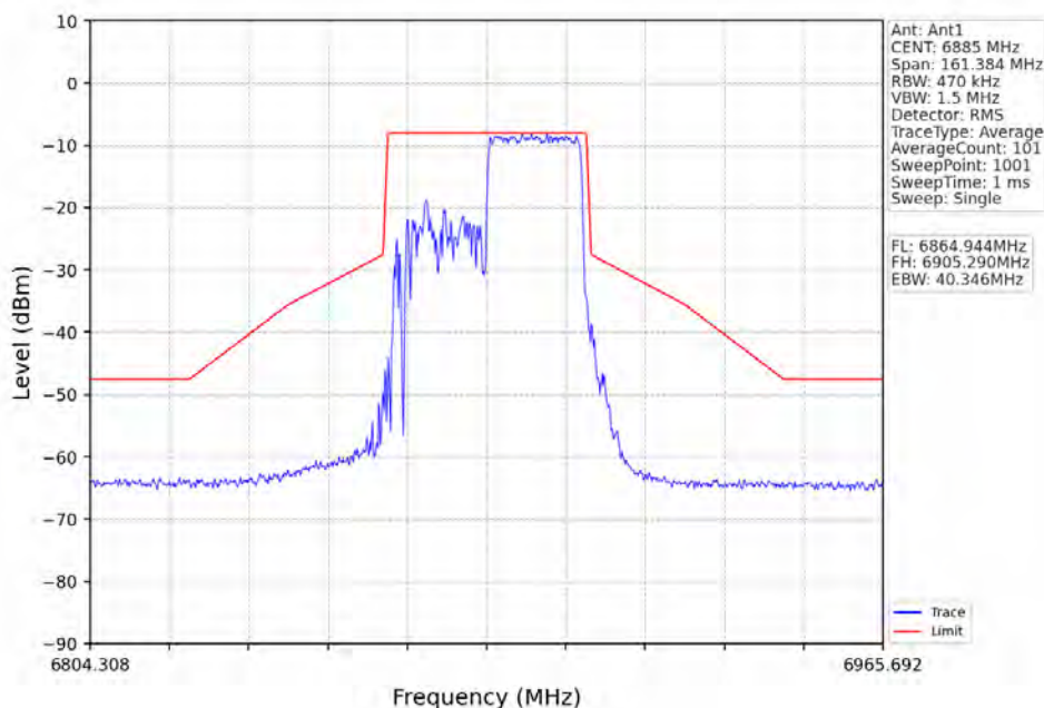
802.11ax(HEW40)_HCH_6885MHz_RU484_Left_Ant1_NTNV
