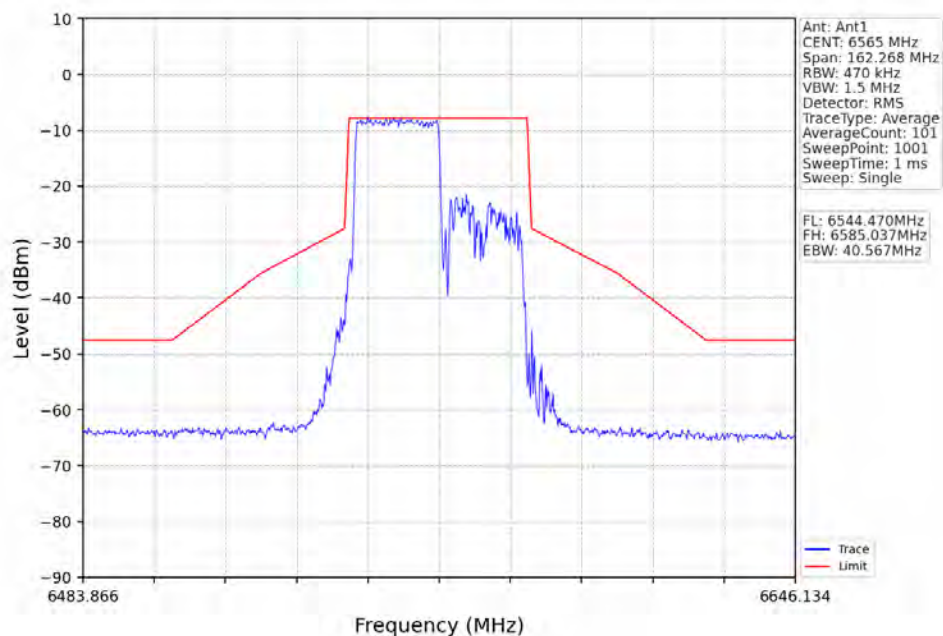
802.11ax(HEW40)_LCH_6565MHz_RU242_Left_Ant1_NTNV
