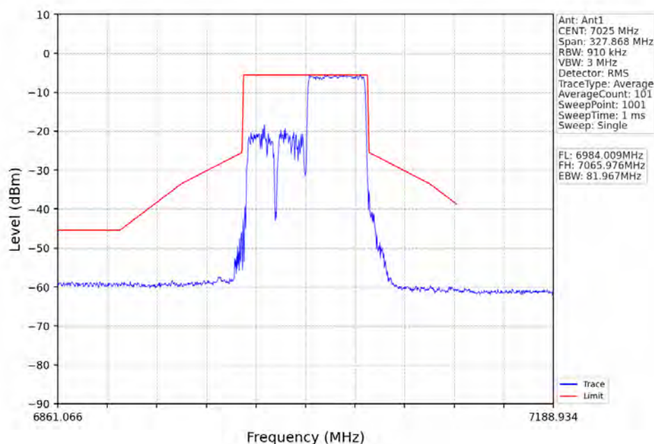
802.11ax(HEW80)_HCH_7025MHz_RU996_Left_Ant1_NTNV
