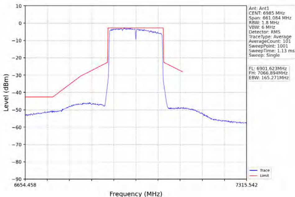
802.11ax(HEW160)_MCH_6985MHz_2xRU996_Left_Ant1_NTNV
