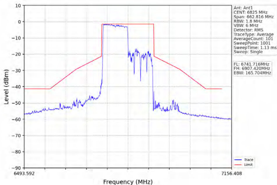
802.11ax(HEW160)_HCH_6825MHz_RU996_Left_Ant1_NTNV
