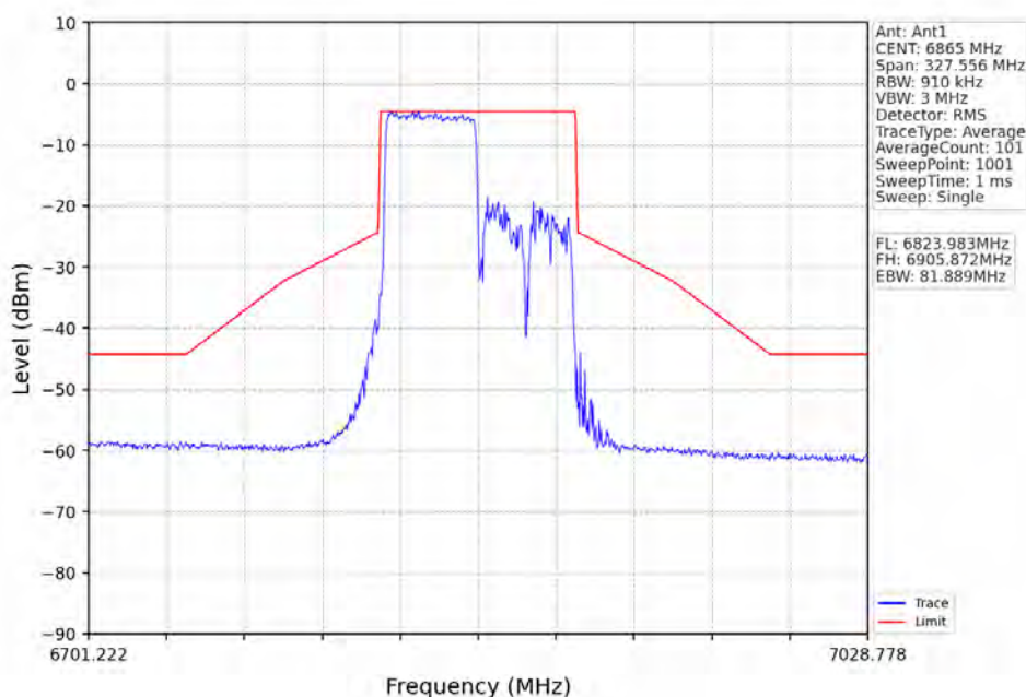
802.11ax(HEW80)_HCH_6865MHz_RU484_Right_Ant1_NTNV
