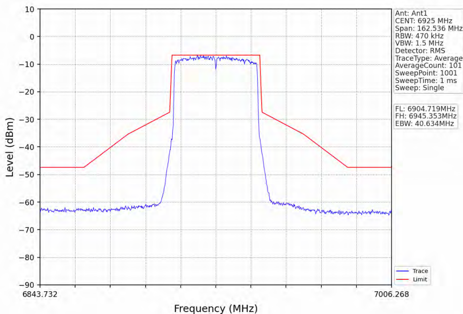
802.11ax(HEW40)_LCH_6925MHz_RU484_Left_Ant1_NTNV
