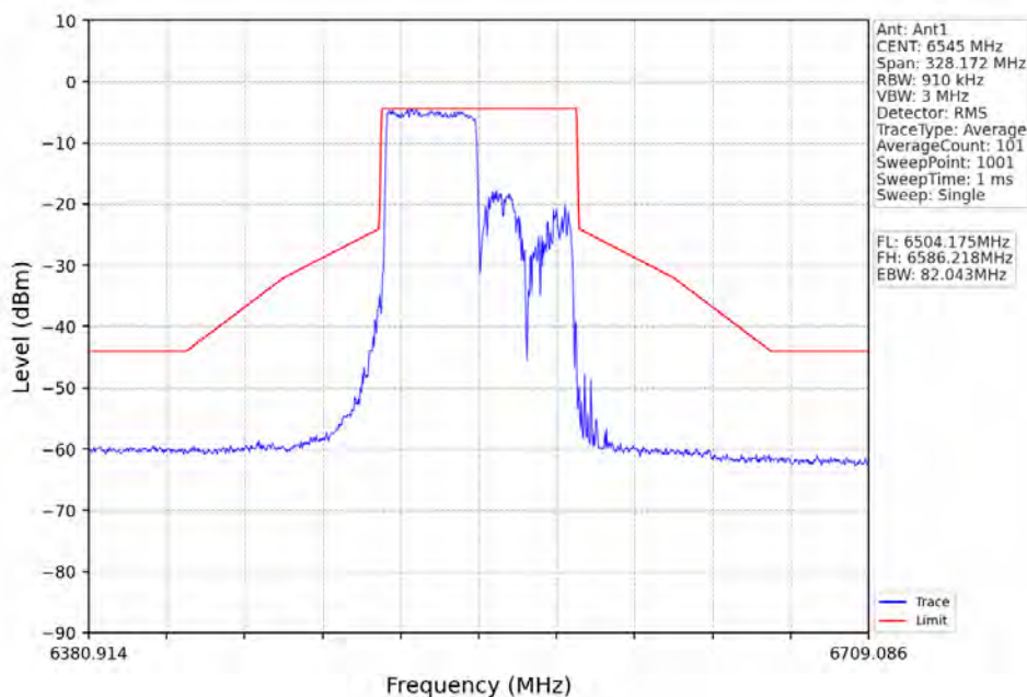
802.11ax(HEW80)_HCH_6545MHz_RU484_Left_Ant1_NTNV
