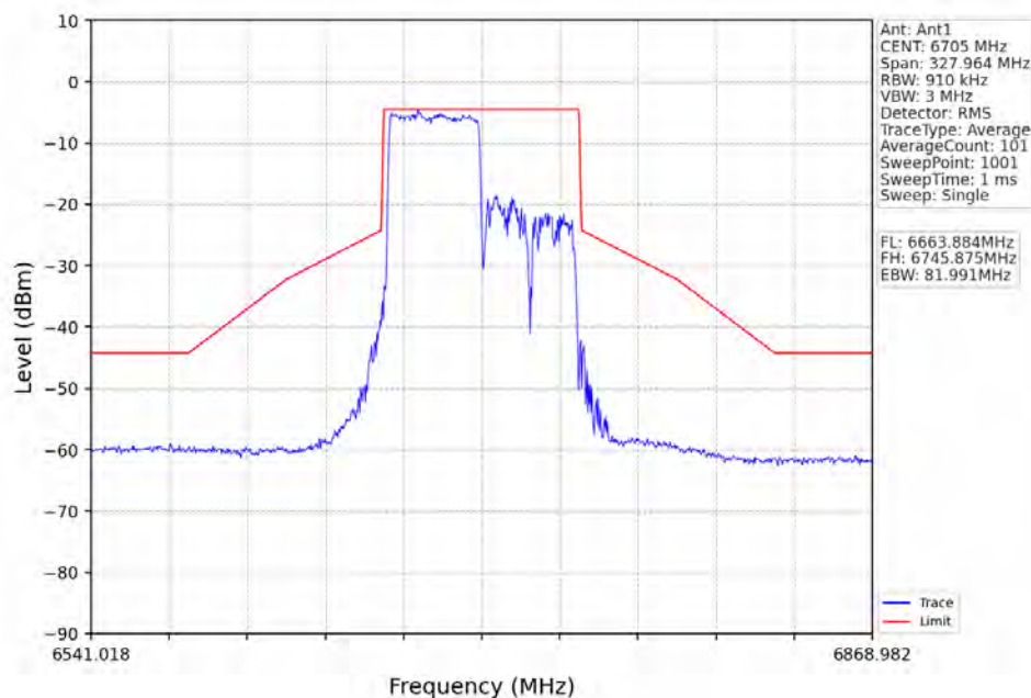
802.11ax(HEW80)_MCH_6705MHz_RU484_Left_Ant1_NTNV
