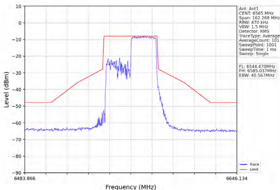
802.11ax(HEW40)_LCH_6565MHz_RU484_Left_Ant1_NTNV
