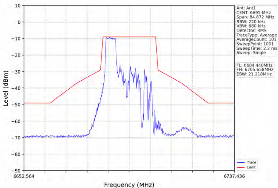
802.11ax(HEW20)_MCH_6695MHz_RU52_Left_Ant1_NTNV
