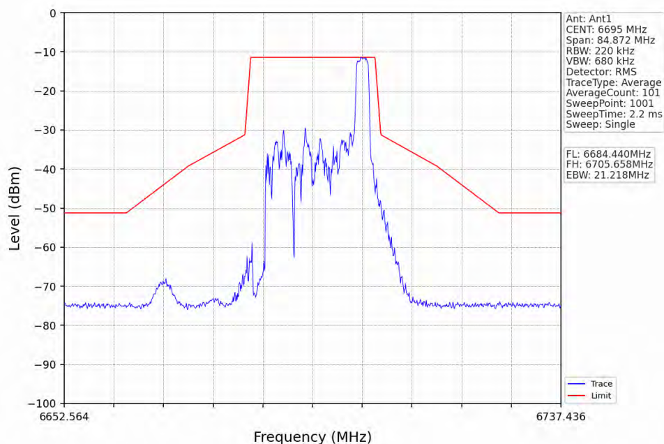
802.11ax(HEW20)_MCH_6695MHz_RU52_Left_Ant1_NTNV
