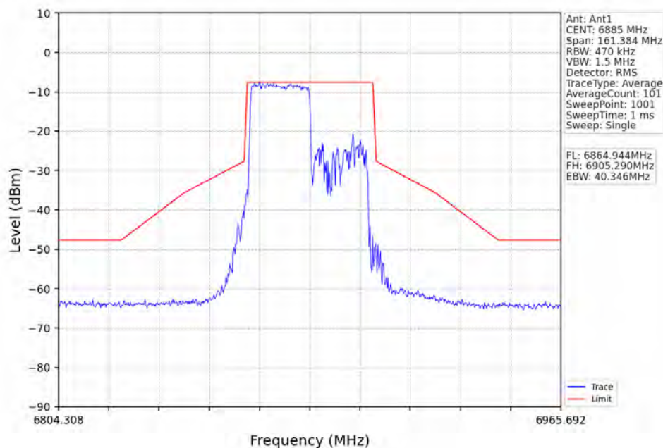
802.11ax(HEW40)_HCH_6885MHz_RU242_Left_Ant1_NTNV
