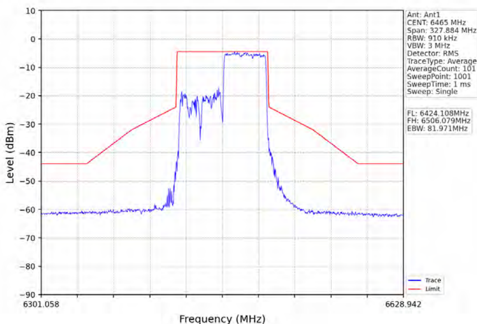
802.11ax(HEW80)_LCH_6465MHz_RU996_Left_Ant1_NTNV
