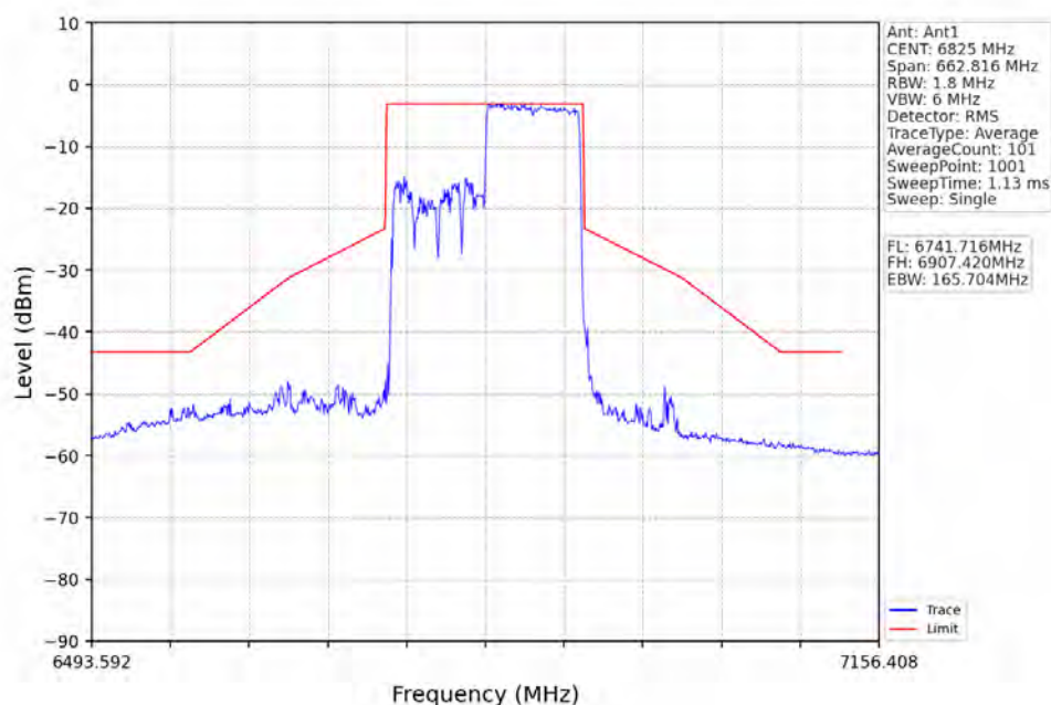
802.11ax(HEW160)_HCH_6825MHz_2xRU996_Left_Ant1_NTNV
