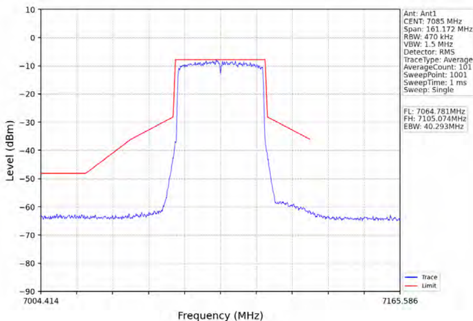
802.11ax(HEW40)_HCH_7085MHz_RU484_Left_Ant1_NTNV
