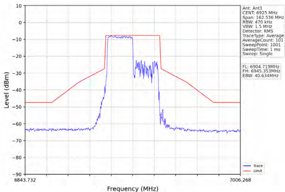
802.11ax(HEW40)_LCH_6925MHz_RU242_Left_Ant1_NTNV
