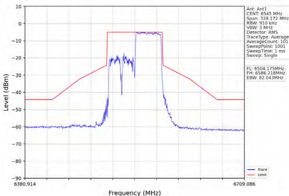
802.11ax(HEW80)_HCH_6545MHz_RU996_Left_Ant1_NTNV
