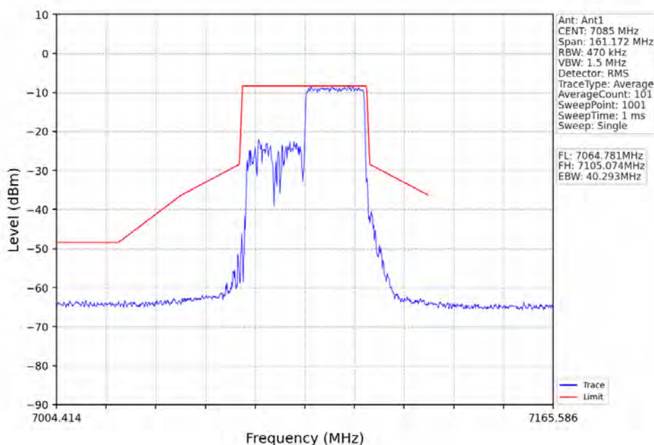
802.11ax(HEW40)_HCH_7085MHz_RU484_Left_Ant1_NTNV
