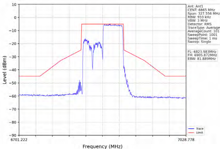
802.11ax(HEW80)_HCH_6865MHz_RU484_Right_Ant1_NTNV
