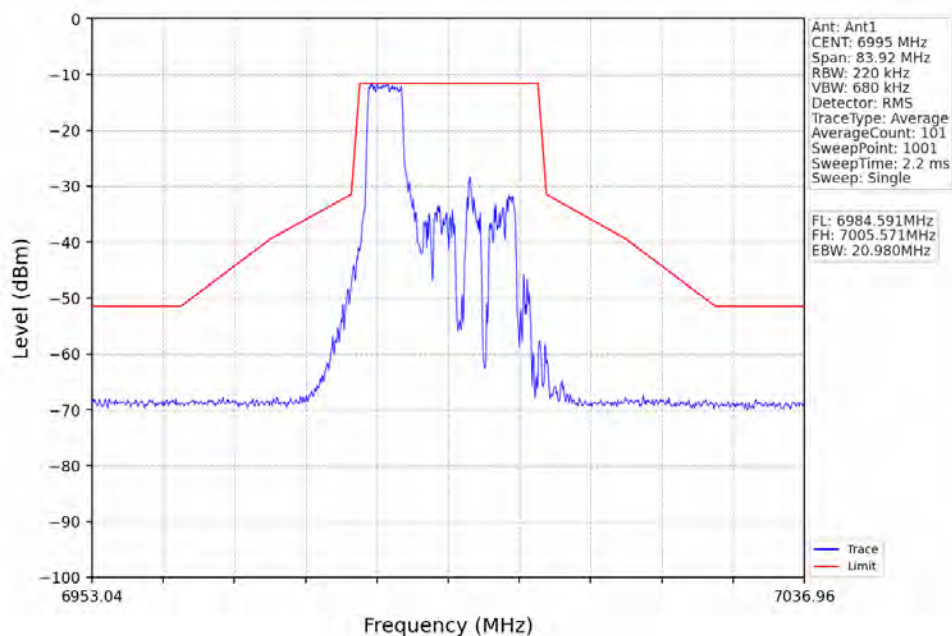
802.11ax(HEW20)_MCH_6995MHz_RU52_Left_Ant1_NTNV
