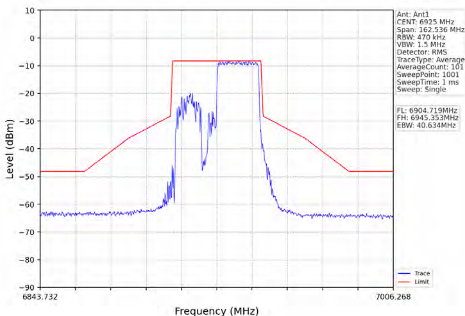
802.11ax(HEW40)_LCH_6925MHz_RU484_Left_Ant1_NTNV
