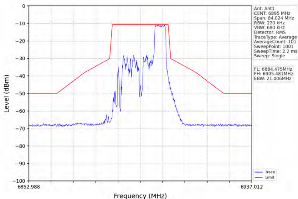
802.11ax(HEW20)_LCH_6895MHz_RU52_Right_Ant1_NTNV
