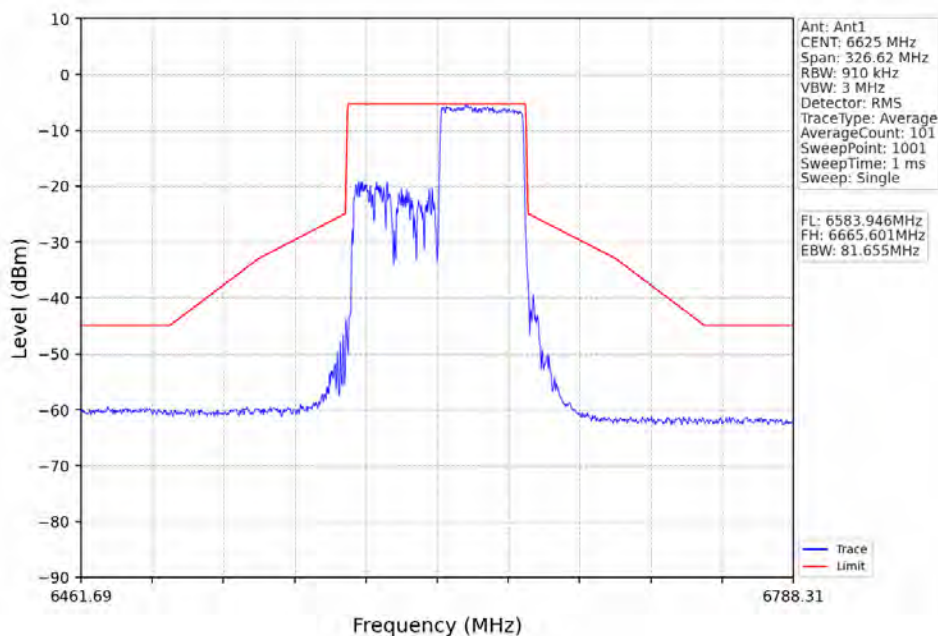
802.11ax(HEW80)_LCH_6625MHz_RU484_Right_Ant1_NTNV
