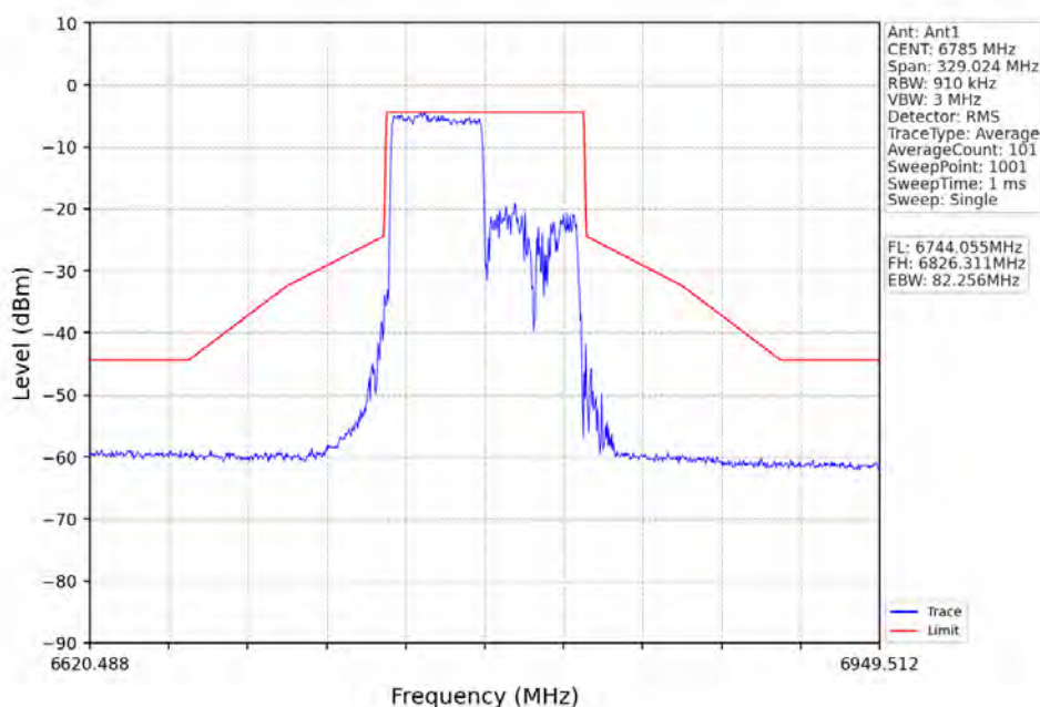
802.11ax(HEW80)_HCH_6785MHz_RU484_Right_Ant1_NTNV
