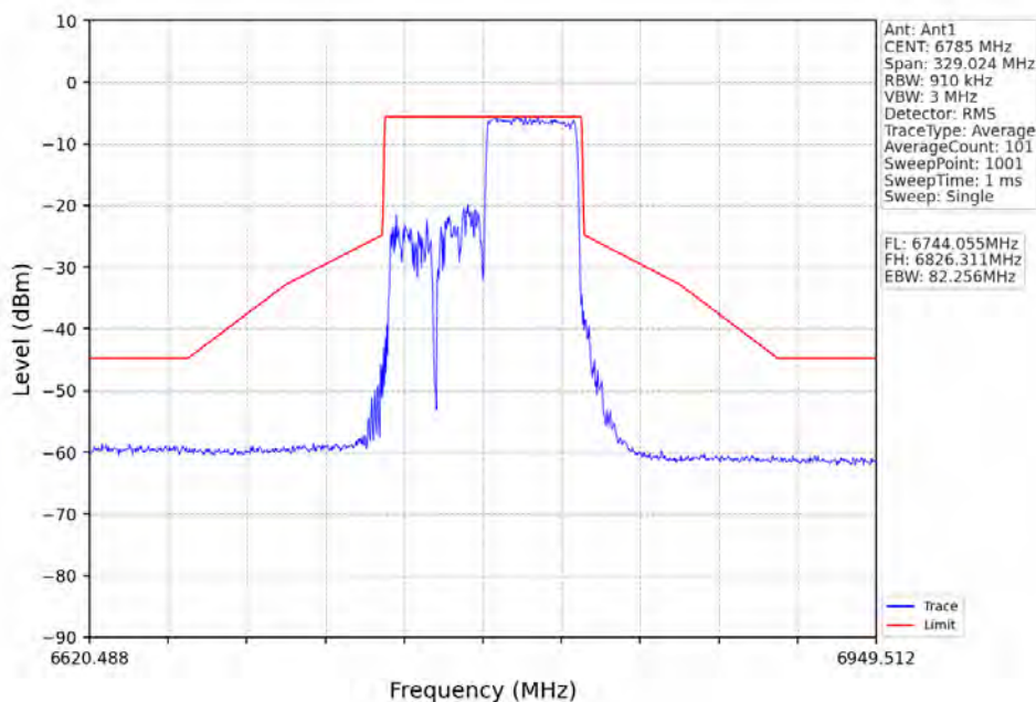
802.11ax(HEW80)_HCH_6785MHz_RU484_Right_Ant1_NTNV
