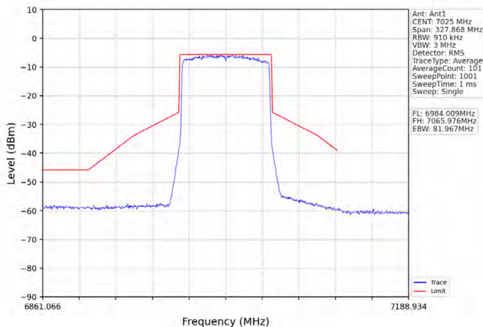
802.11ax(HEW80)_HCH_7025MHz_RU996_Left_Ant1_NTNV
