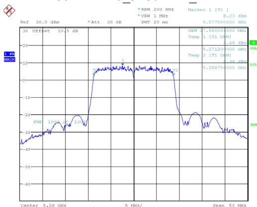
802.11ac20_5280MHz_Chain 1
