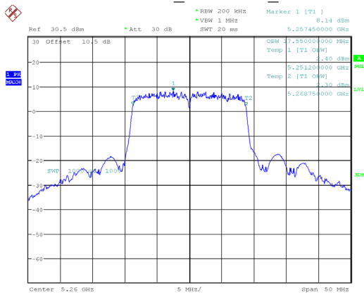
802.11ac20_5260MHz_Chain 0
