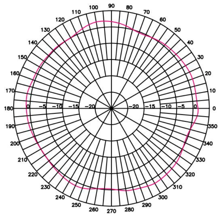
H-Plane Pattern @ 2.45GHz
