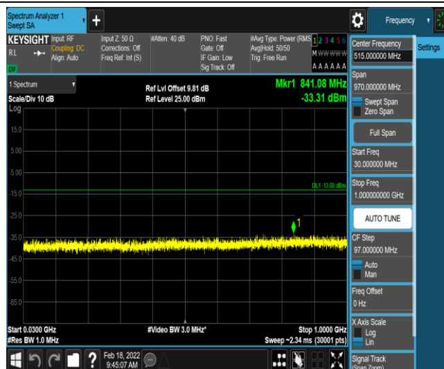
Band2-20MHz-QPSK-18700-1-0-Low-30-1000--33.31-PASS
