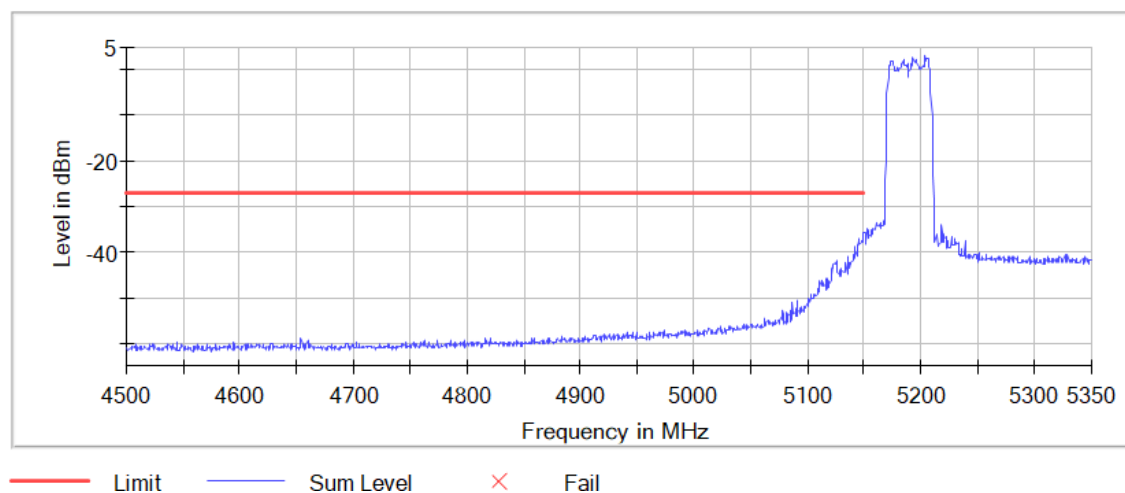
Band Edge
