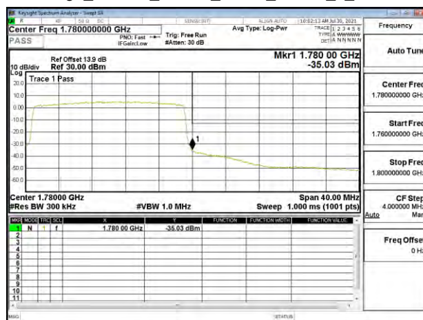
Band Edge_Band66_20MHz_QPSK_RB100_0_CH132572
