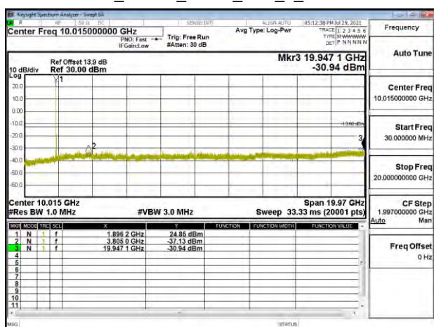
Band2_15MHz_QPSK_RB1_0_CH19125
