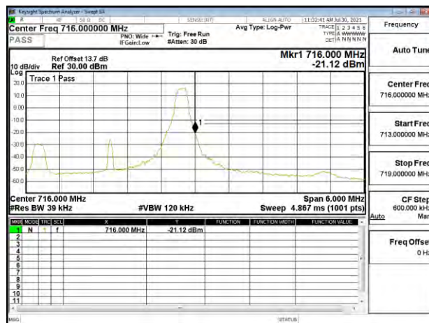
Band Edge_Band12_3MHz_QPSK_RB1_14_CH23165
