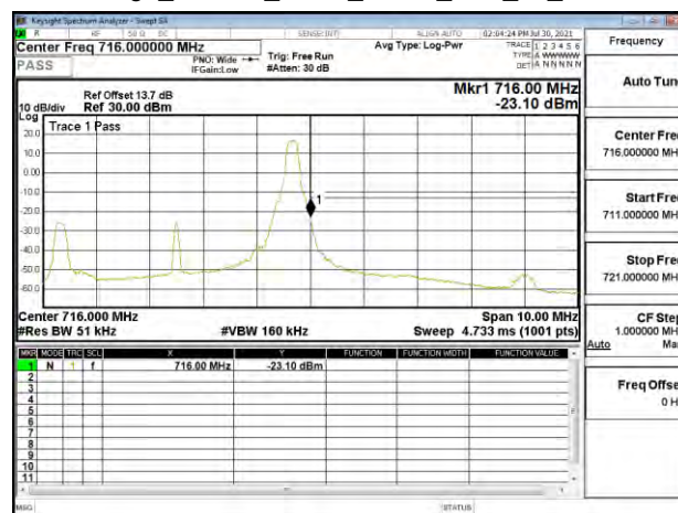
Band Edge_Band17_5MHz_QPSK_RB1_24_CH23825
