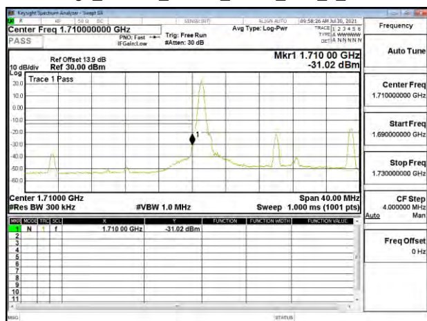
Band Edge_Band66_20MHz_QPSK_RB1_0_CH132072
