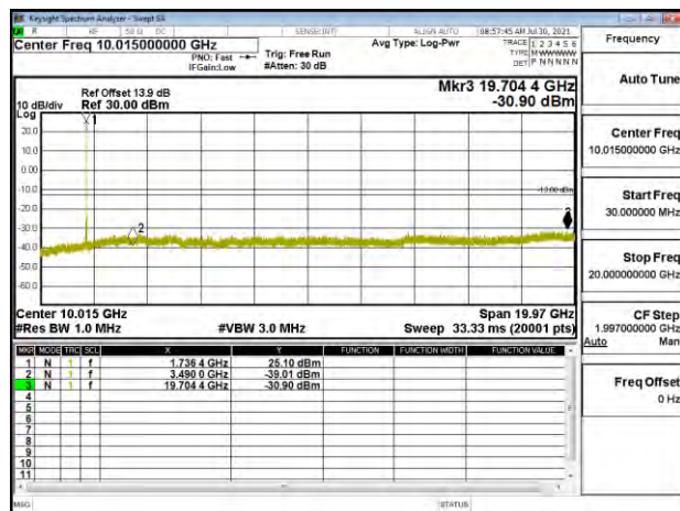
Band4_20MHz_QPSK_RB1_0_CH20300
