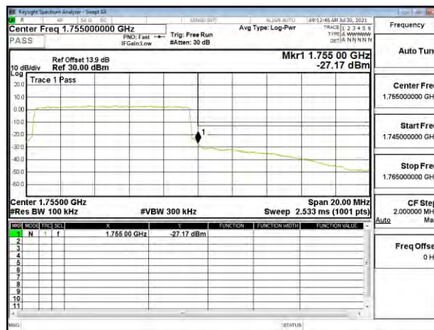
Band Edge_Band4_10MHz_QPSK_RB50_0_CH20350
