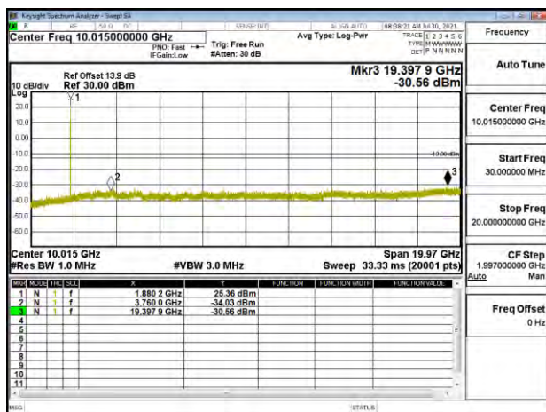
Band2_1.4MHz_QPSK_RB1_0_CH18900
