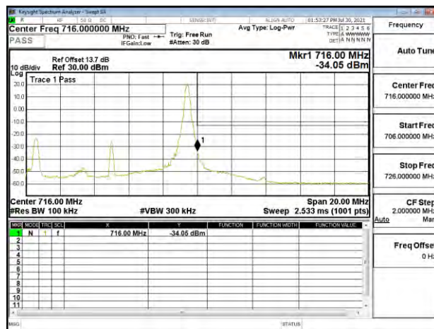
Band Edge_Band17_10MHz_QPSK_RB1_49_CH23800
