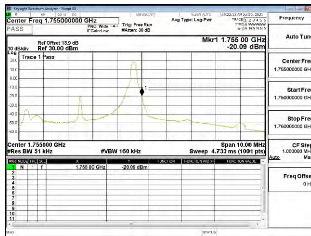
Band Edge_Band4_5MHz_QPSK_RB1_24_CH20375
