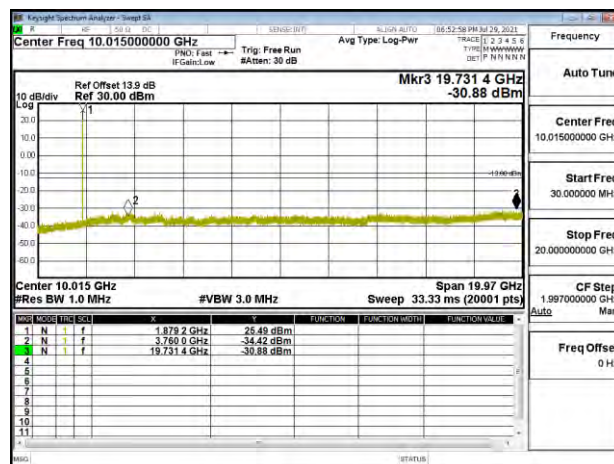
Band2_3MHz_QPSK_RB1_0_CH18900
