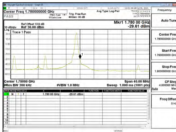
Band Edge_Band66_20MHz_QPSK_RB1_99_CH132572
