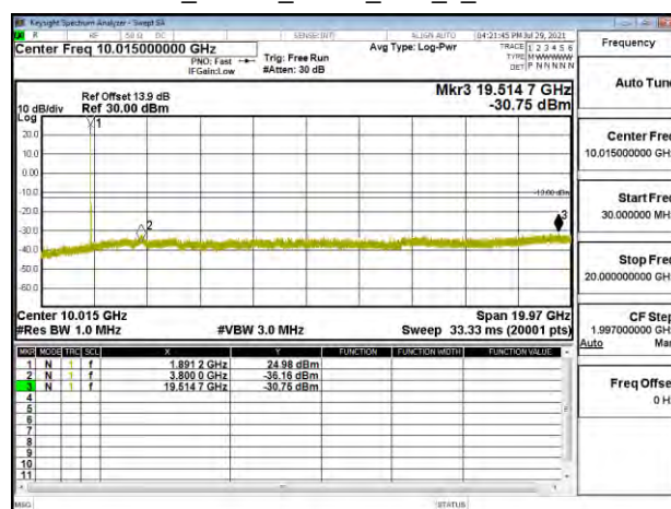
Band2_20MHz_QPSK_RB1_0_CH19100
