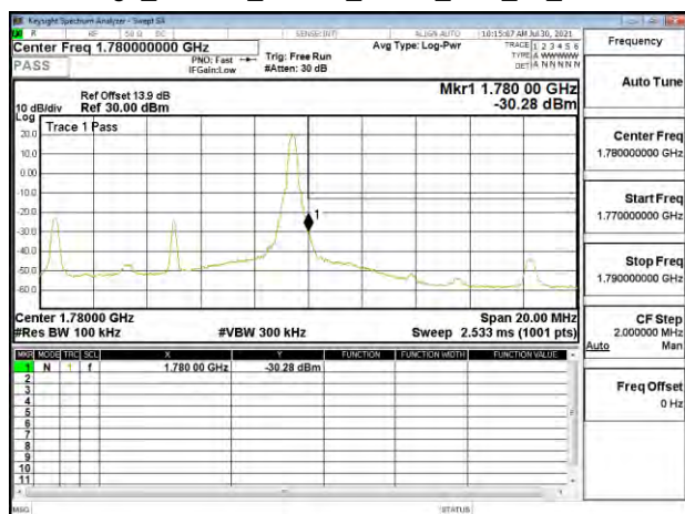
Band Edge_Band66_10MHz_QPSK_RB1_49_CH132622
