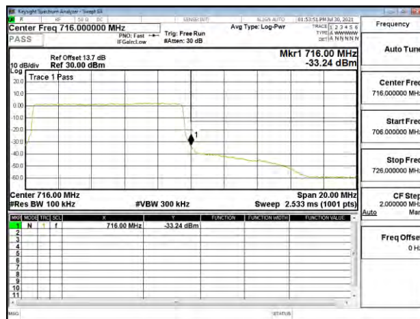
Band Edge_Band17_10MHz_QPSK_RB50_0_CH23800
