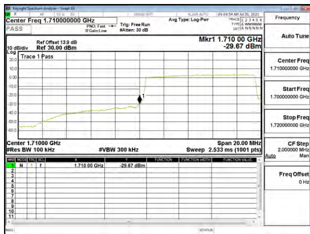
Band Edge_Band4_10MHz_QPSK_RB50_0_CH20000
