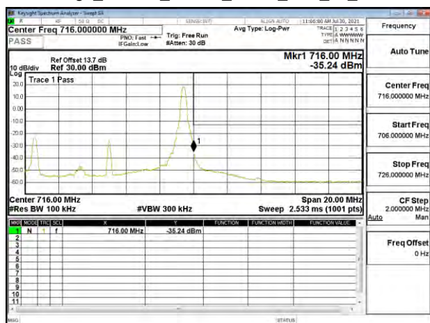
Band Edge_Band12_10MHz_QPSK_RB1_49_CH23130
