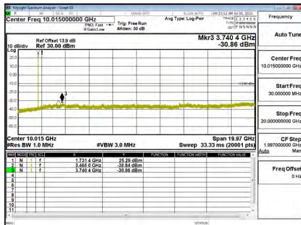
Band4_3MHz_QPSK_RB1_0_CH20175
