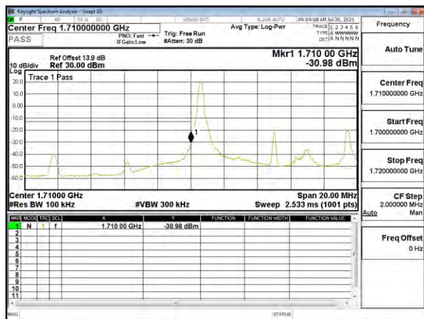
Band Edge_Band4_10MHz_QPSK_RB1_0_CH20000
