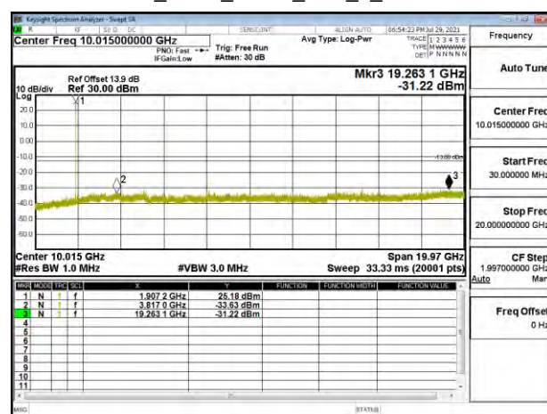
Band2_3MHz_QPSK_RB1_0_CH19185
