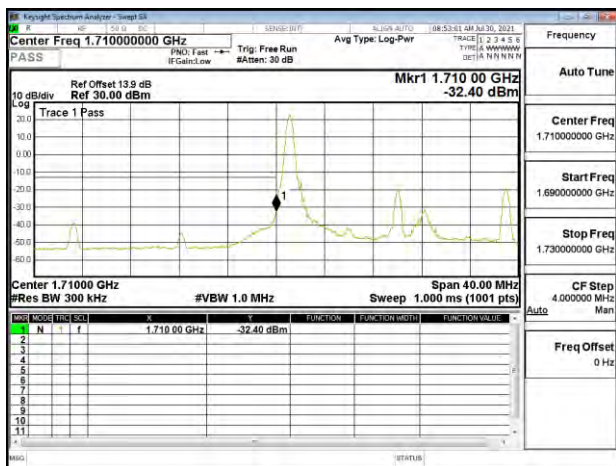
Band Edge_Band4_20MHz_QPSK_RB1_0_CH20050
