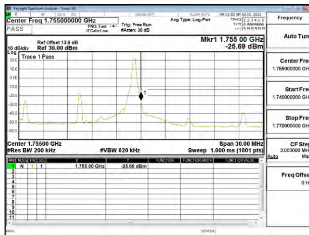
Band Edge_Band4_15MHz_QPSK_RB1_74_CH20325
