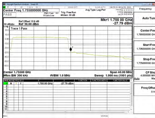
Band Edge_Band4_20MHz_QPSK_RB100_0_CH20300
