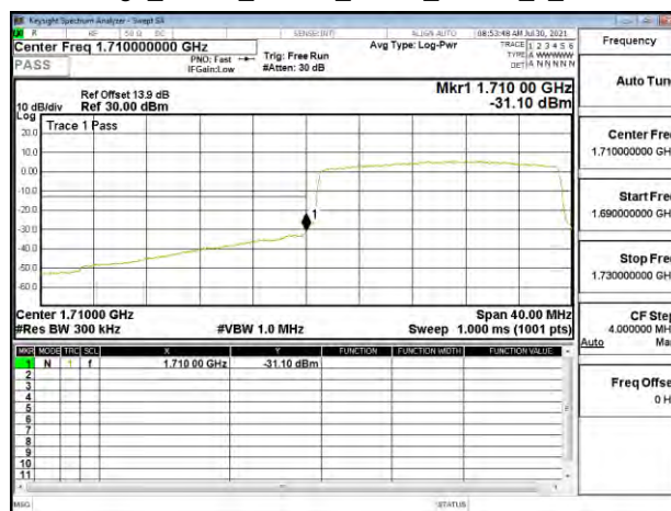
Band Edge_Band4_20MHz_QPSK_RB100_0_CH20050
