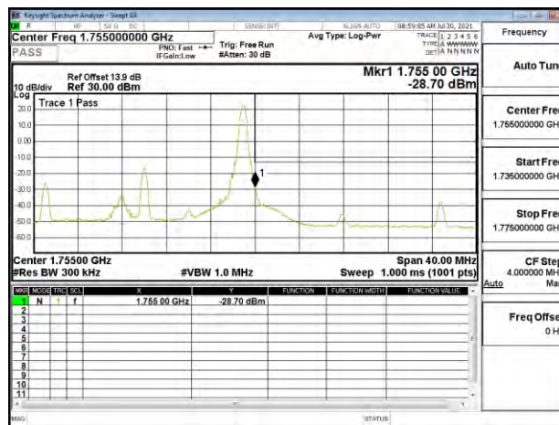
Band Edge_Band4_20MHz_QPSK_RB1_99_CH20300
