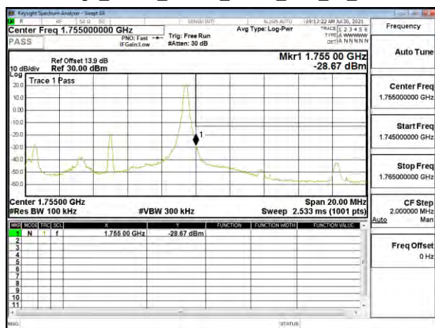
Band Edge_Band4_10MHz_QPSK_RB1_49_CH20350
