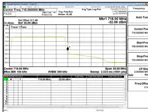
Band Edge_Band12_10MHz_QPSK_RB50_0_CH23130
