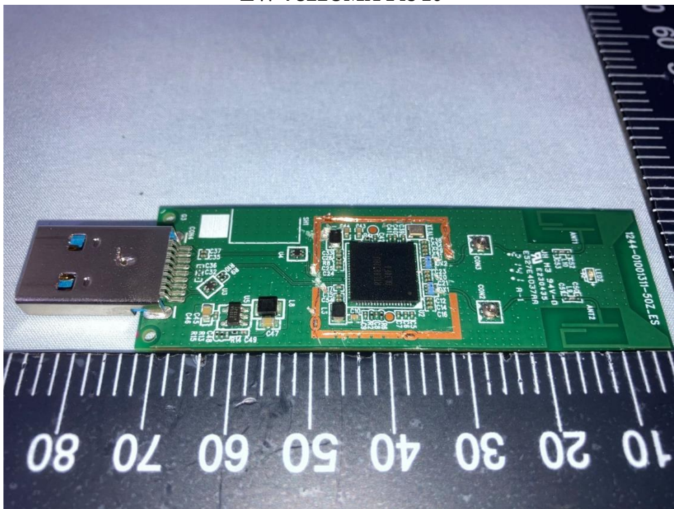
EW-7822UMX Pic 10
