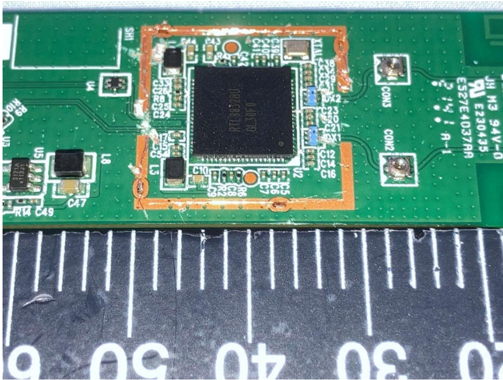
EW-7822UMX Pic 11
