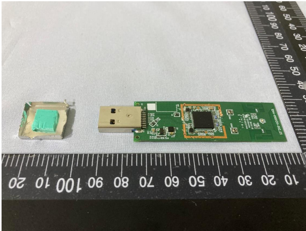
EW-7822UMX Pic 9
