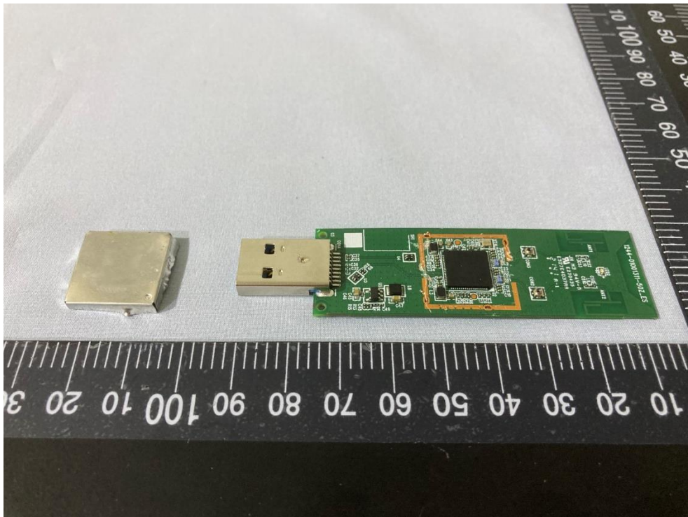
EW-7822UMX Pic 8
