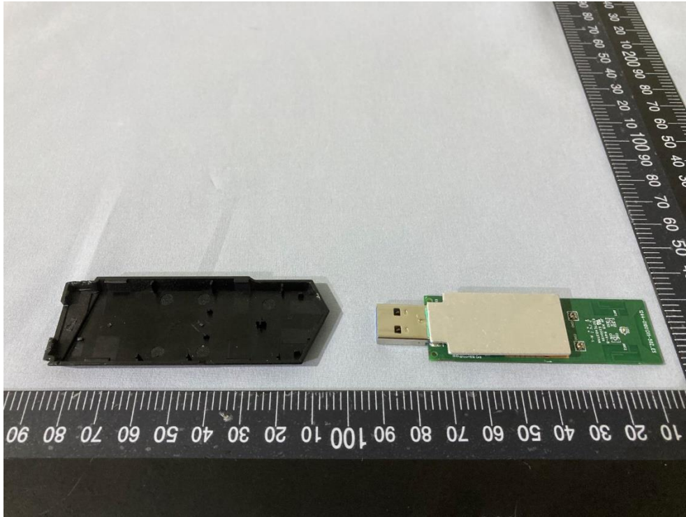
EW-7822UMX Pic 3
