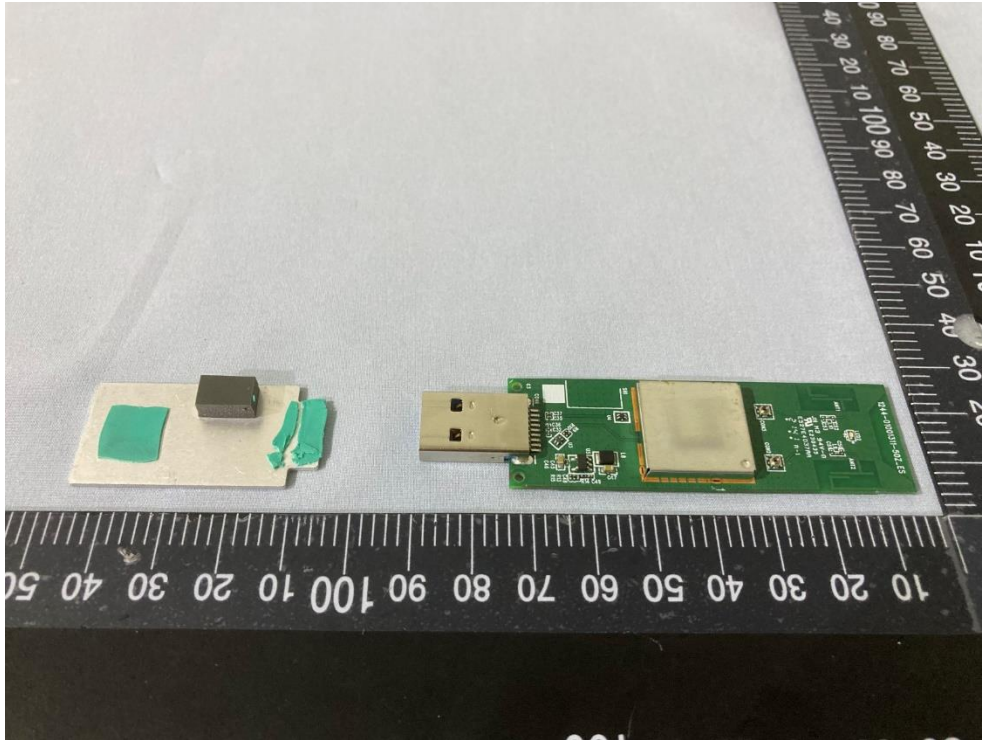
EW-7822UMX Pic 7
