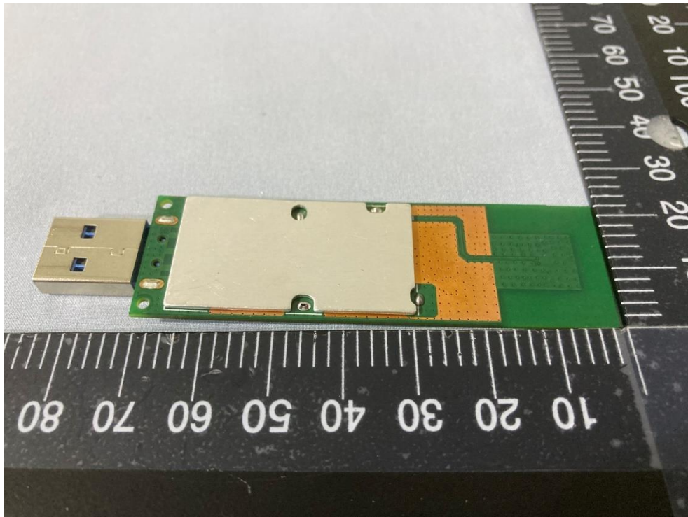
EW-7822UMX Pic 12
