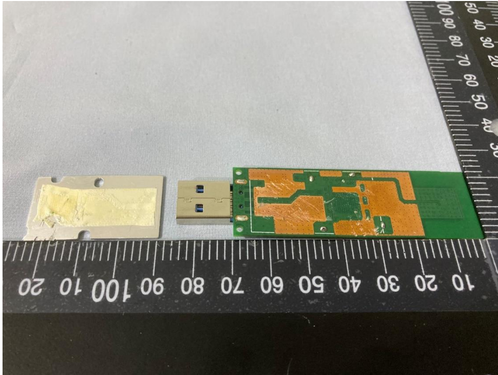
EW-7822UMX Pic 13
