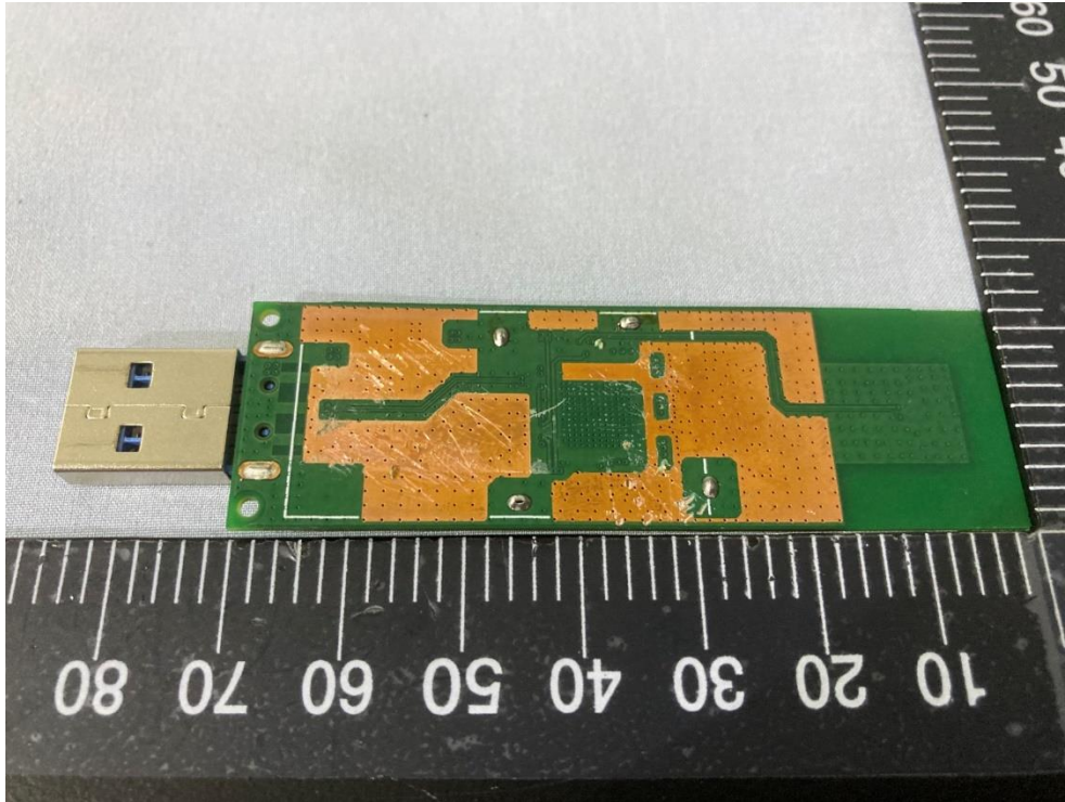
EW-7822UMX Pic 15
