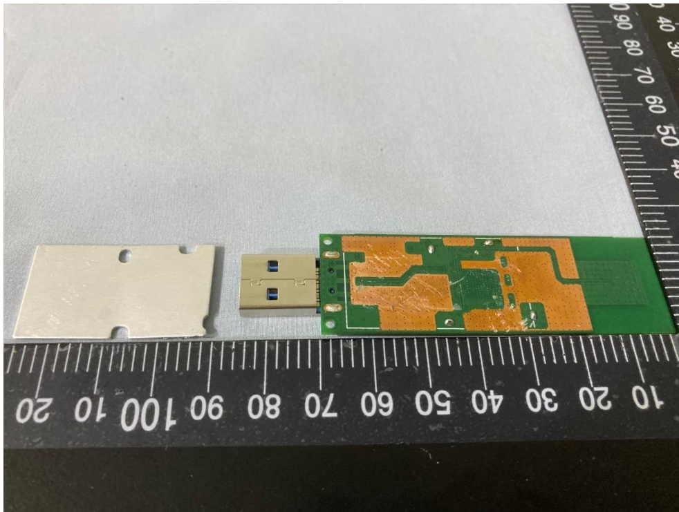
EW-7822UMX Pic 14
