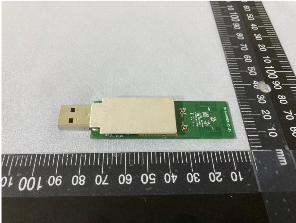
EW-7822UMX Pic 5
