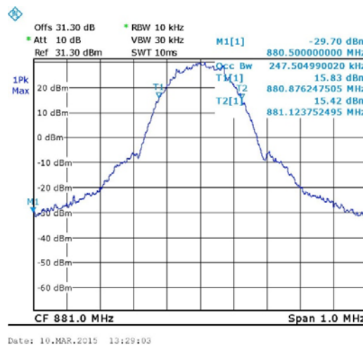
Figure 27. — GSM - Input 881.0 MHz
