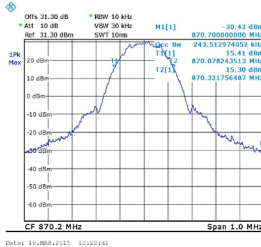
Figure 25. — GSM - Input 870.20MHz
