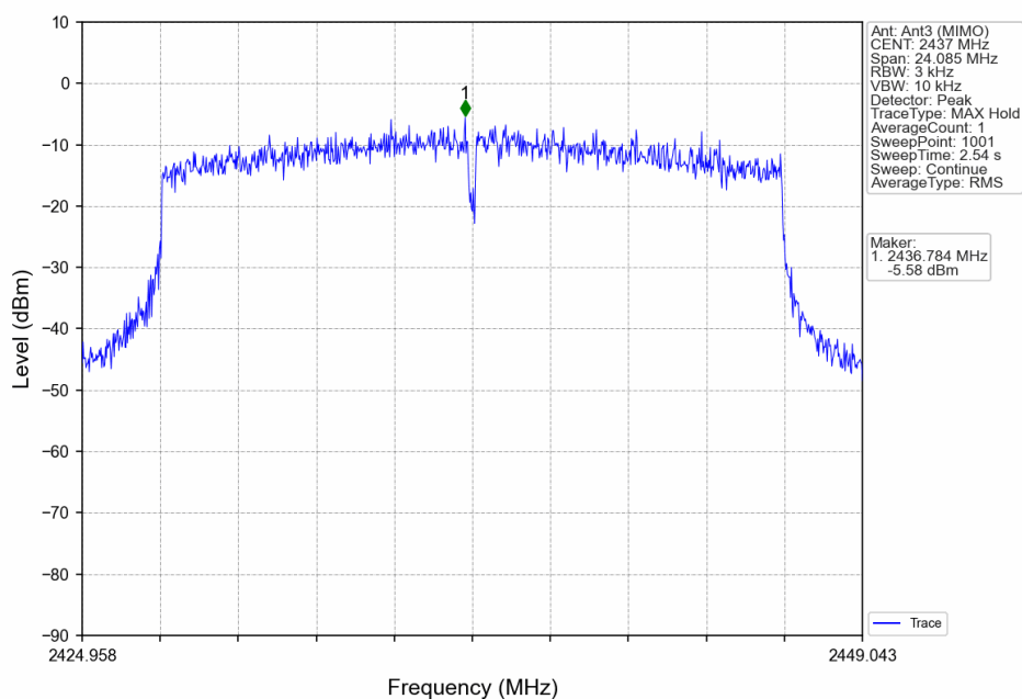
802.11ax(HEW20)_MCH_2437MHz_RU242_Left_Ant3 (MIMO)_NTNV
