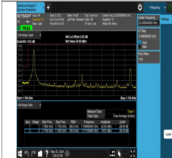
Band66_20MHz_QPSK_132072_1RB#0
