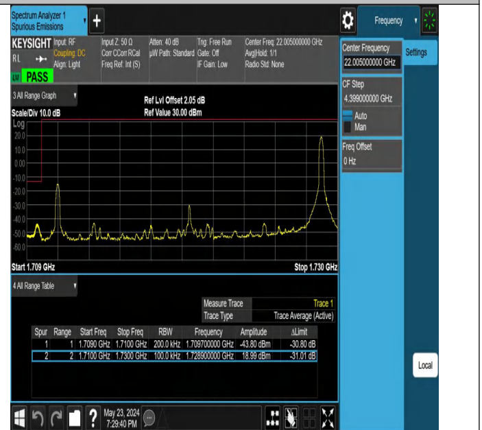
Band66_20MHz_QPSK_132072_1RB#99
