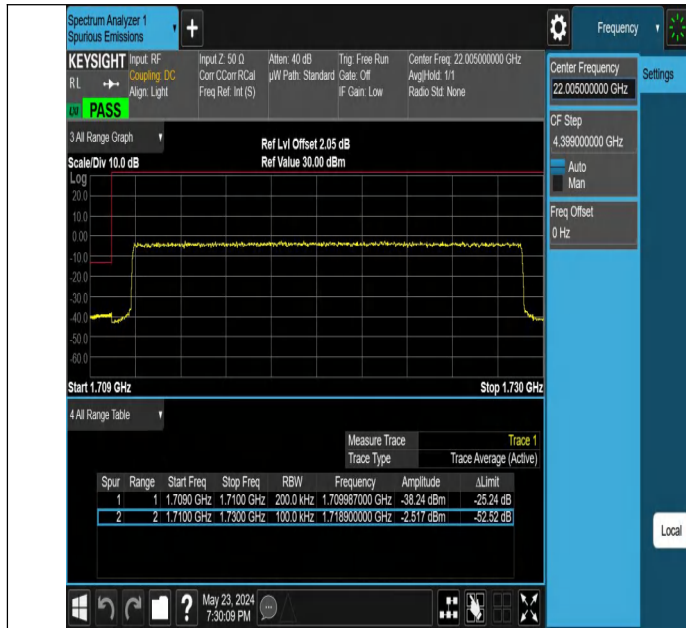
Band66_20MHz_QPSK_132072_100RB#0
