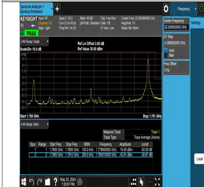
Band66_20MHz_QPSK_132572_1RB#99
