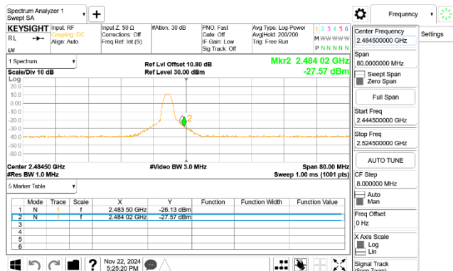
CBE_BLE_1M_2480MHz
