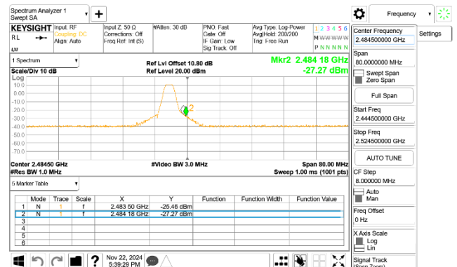
CBE_BLE_2M_2480MHz
