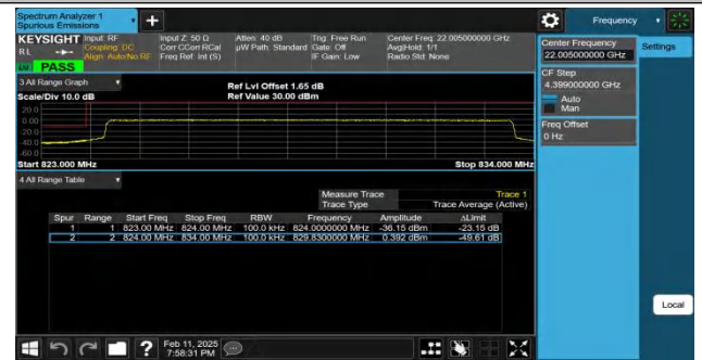
Band26(824-849)-10MHz-QPSK-26840-50RB#0-PASS
