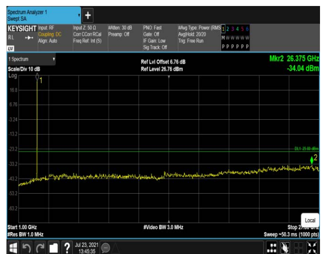
Band38-5MHz-QPSK-38225:1000~27000MHz
