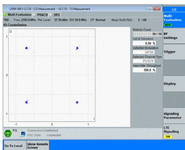
Band41-20MHz-QPSK-40640-100RB#0
