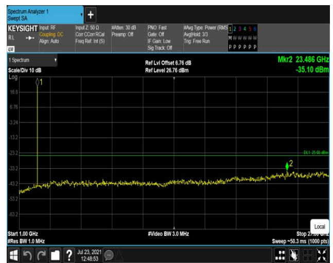
Band7-5MHz-QPSK-21425:1000~27000MHz
