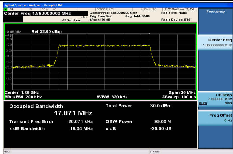
Band2-20MHz-16QAM-18700-100RB#0-17.871
