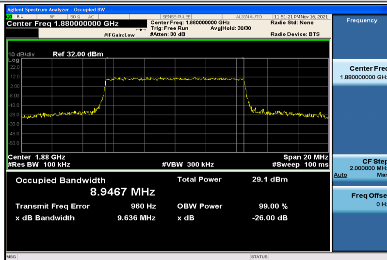
Band2-10MHz-16QAM-18900-50RB#0-8.9467
