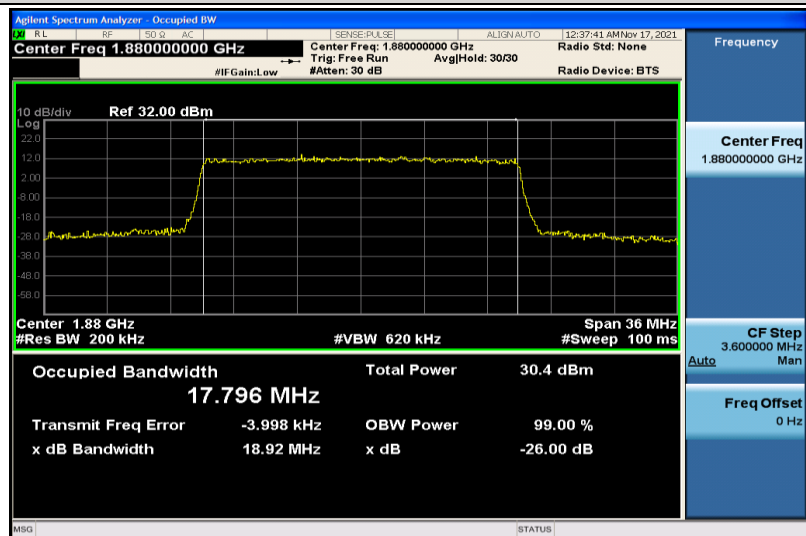
Band2-20MHz-QPSK-18900-100RB#0-17.796
