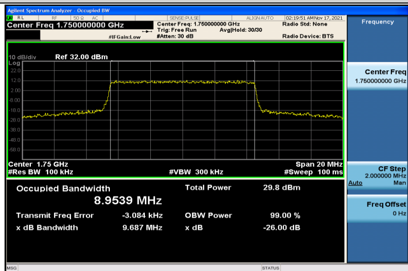
Band4-10MHz-QPSK-20350-50RB#0-8.9539
