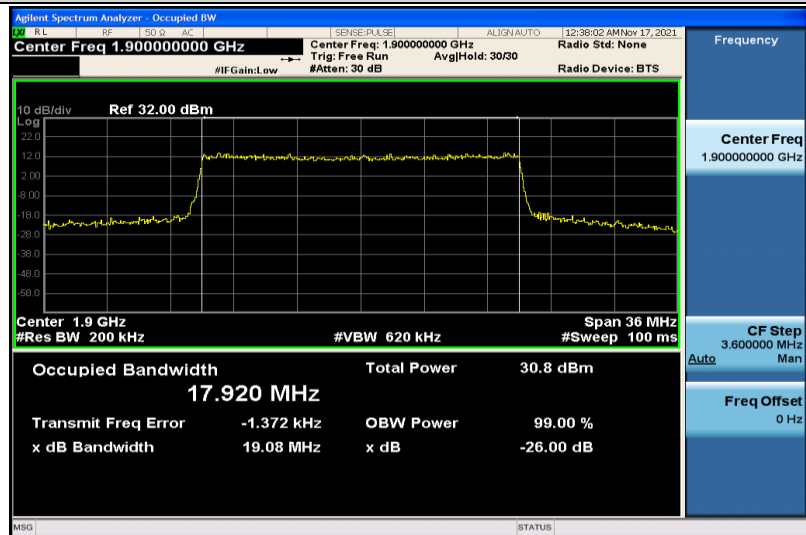
Band2-20MHz-QPSK-19100-100RB#0-17.920
