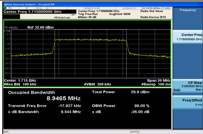
Band4-10MHz-QPSK-20000-50RB#0-8.9465
