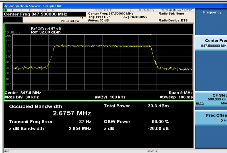
Band5-3MHz-QPSK-20635-15RB#0-2.6757
