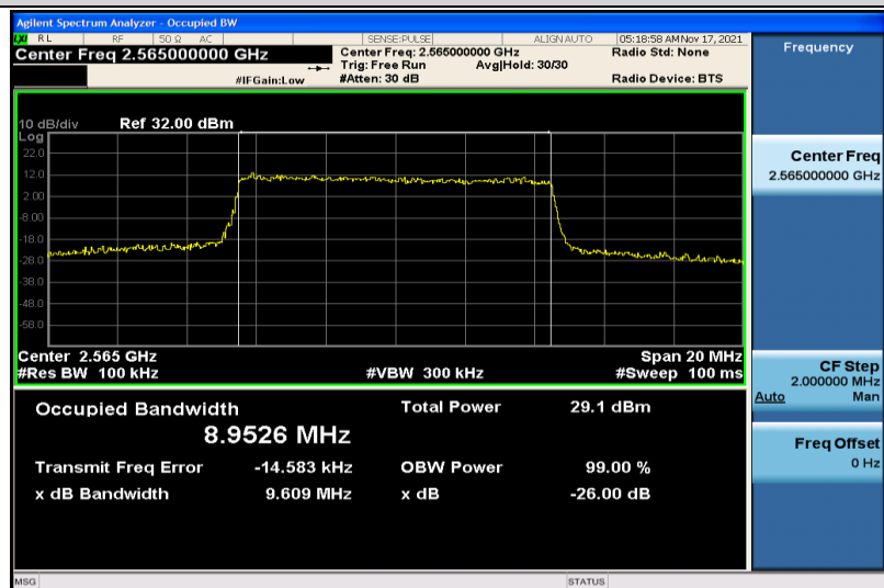
Band7-10MHz-QPSK-21400-50RB#0-8.9526
