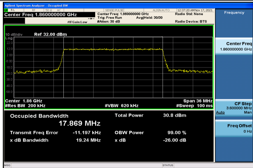
Band2-20MHz-QPSK-18700-100RB#0-17.869
