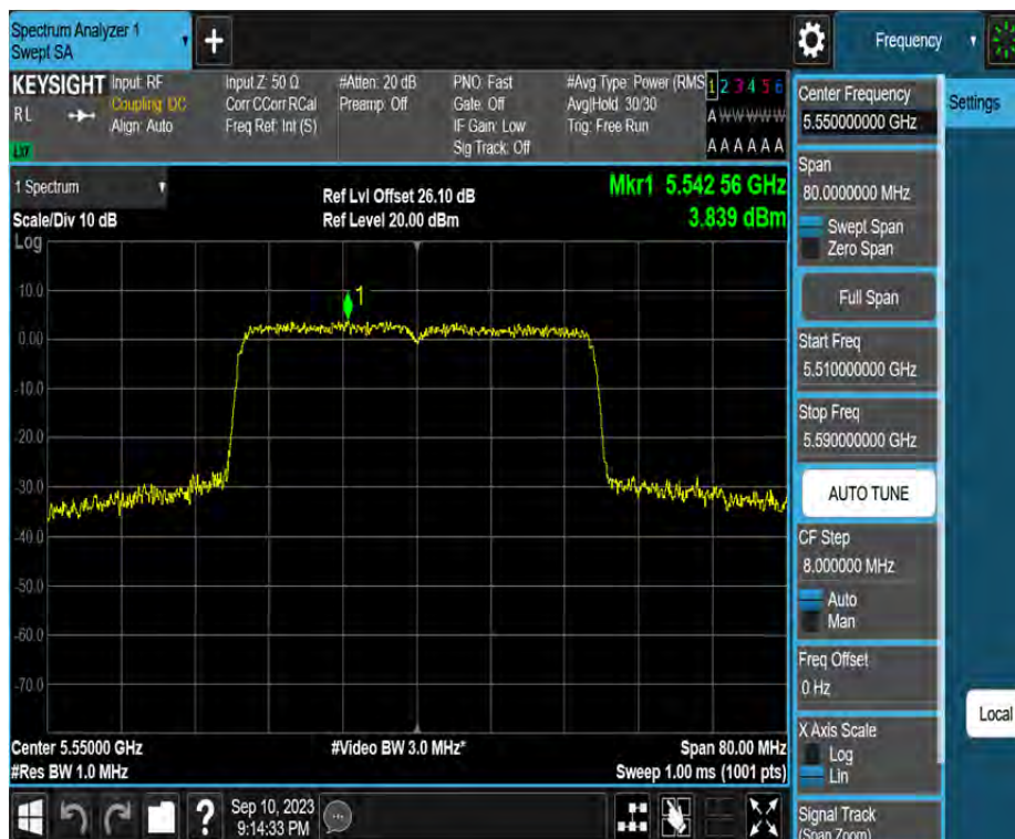
11AX40MIMO_Ant4_5550
