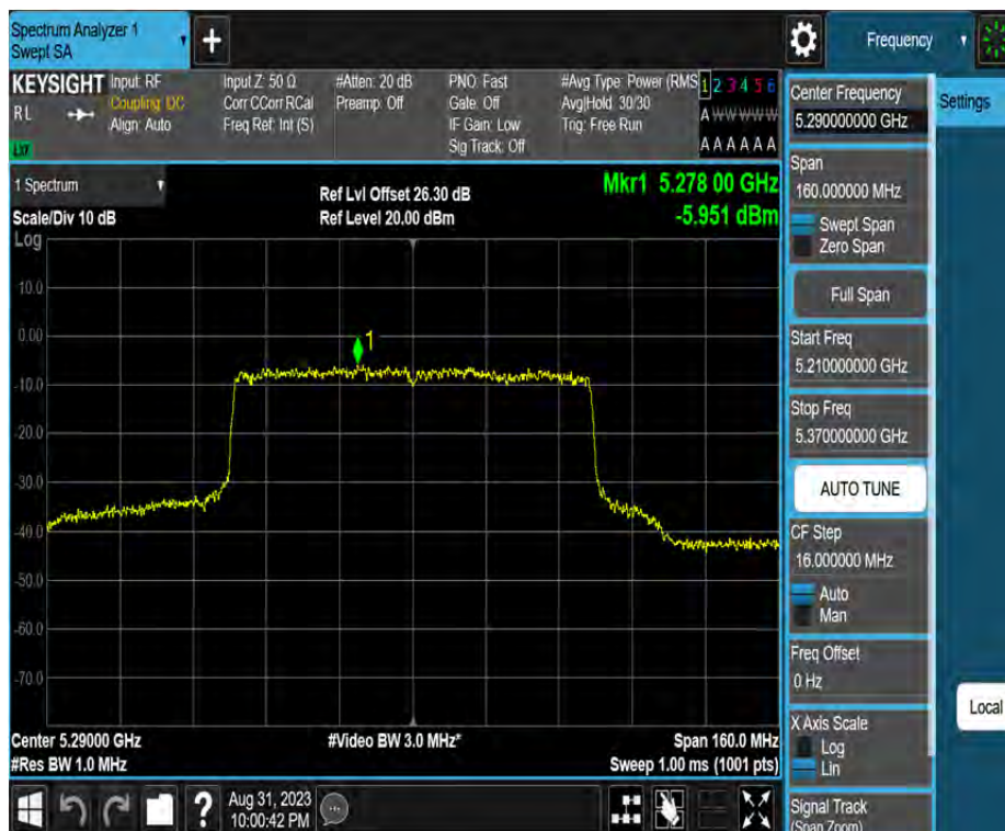
11AX80MIMO_Ant4_5290
