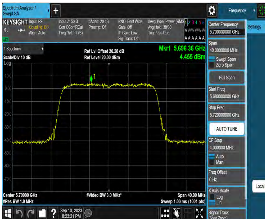
11AX20MIMO_Ant4_5700
