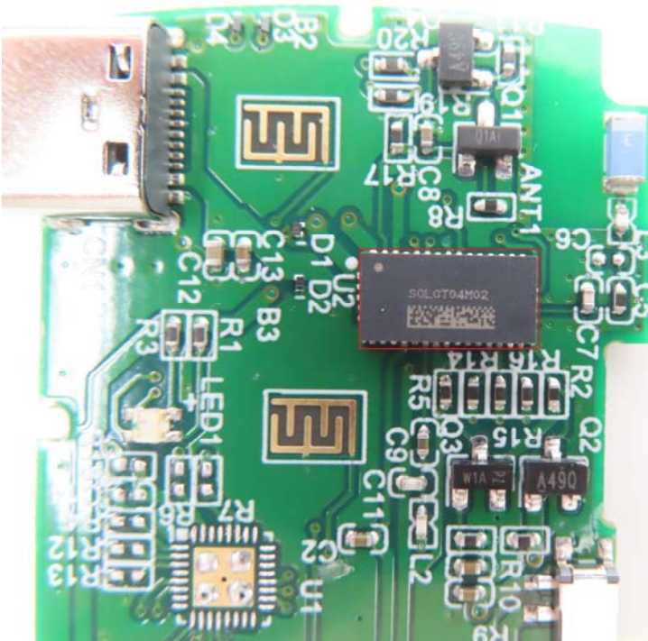
RF IC
