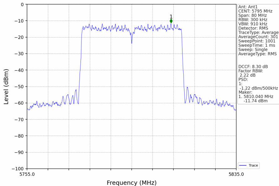
802.11ax(HEW40)_HCH_5795MHz_RU484_Left_Ant1_NTNV
