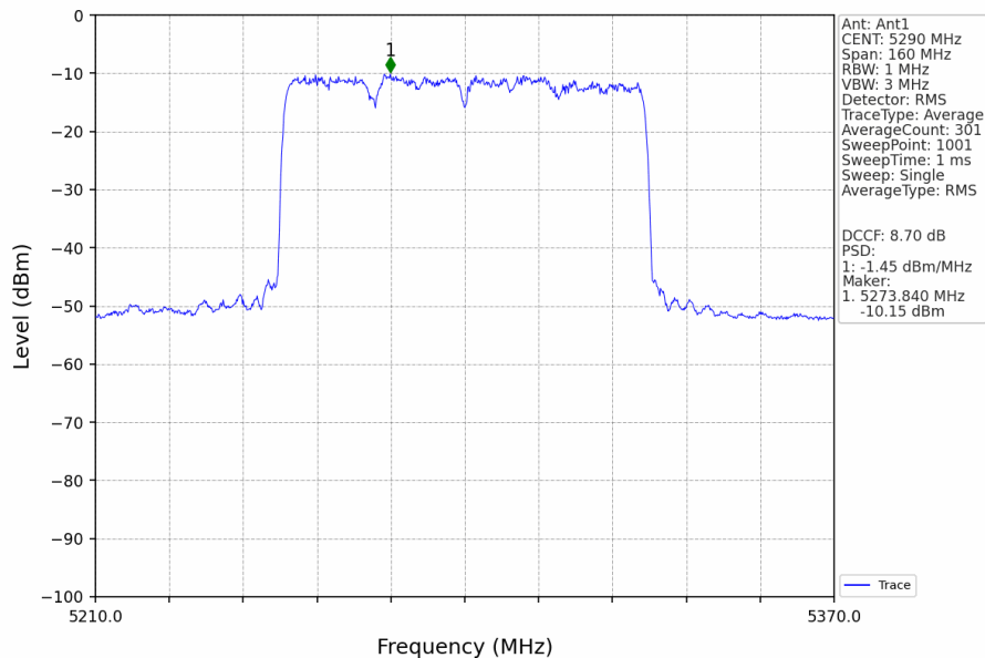
802.11ax(HEW80)_MCH_5290MHz_RU996_Left_Ant1_NTNV
