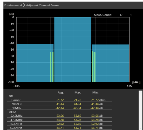
90MHz_30kHz_3655MHz-OFDM QPSK_RB243@0 -41.34,-42.34dB
