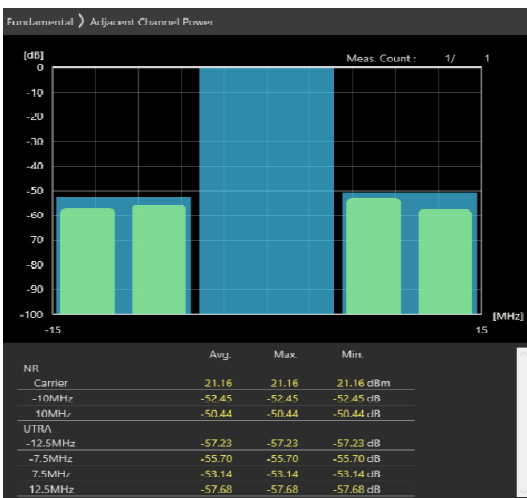
10MHz_30kHz_3695MHz-OFDM QPSK_RB1@23 -52.45,-50.44dB
