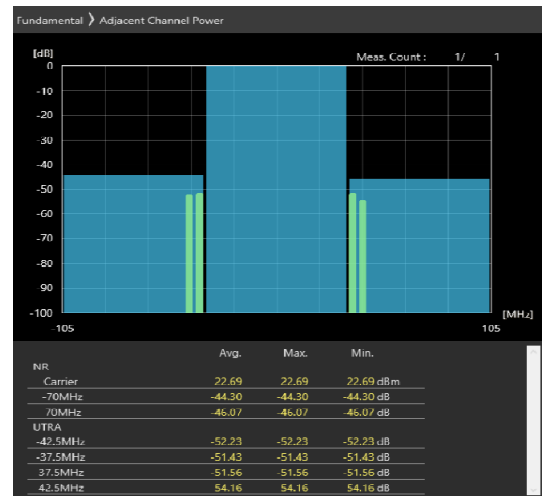
70MHz_30kHz_3665MHz-OFDM QPSK_RB90@45 -44.3,-46.07dB
