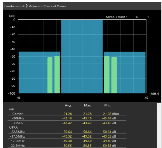
30MHz_30kHz_3685MHz-OFDM QPSK_RB75@0 -43.18,-43.42dB
