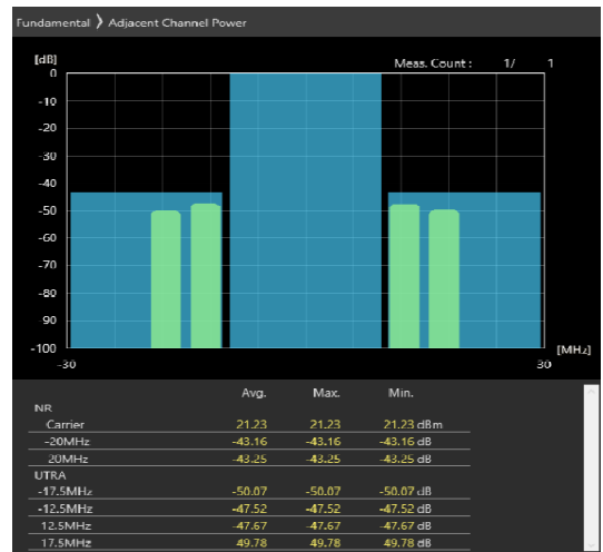
20MHz_30kHz_3690MHz-OFDM QPSK_RB50@0 -43.16,-43.25dB
