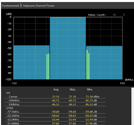
100MHz_30kHz_3650MHz-OFDM QPSK_RB1@272 -45.73,-46.33dB
