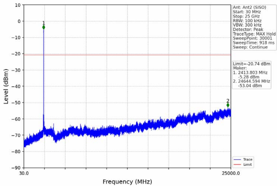
802.11b_LCH_2412MHz_Ant2 (SISO)_NTNV
