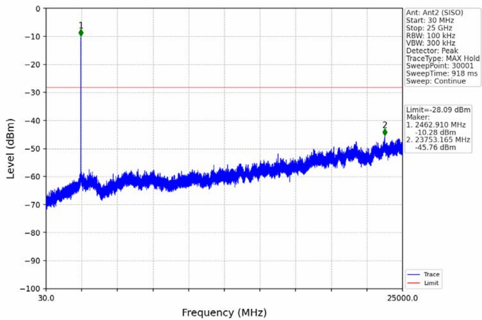
802.11g_HCH_2462MHz_Ant2 (SISO)_NTNV
