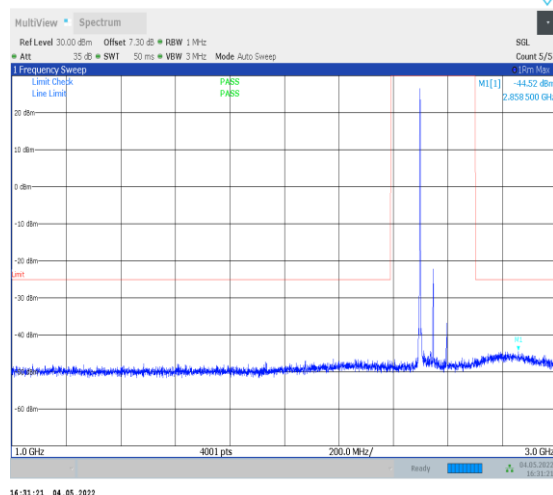
1-N41--30-100-L-1-DFT-PI2BPSK-Inner_1RB_Left-1 @1-1000-3000-Ant0--44.52--25-PASS
