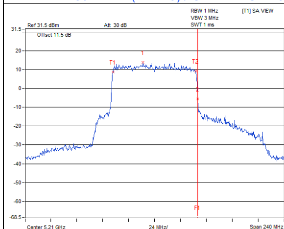
802.11be (EHT80) / Chain 1 : CH 42
